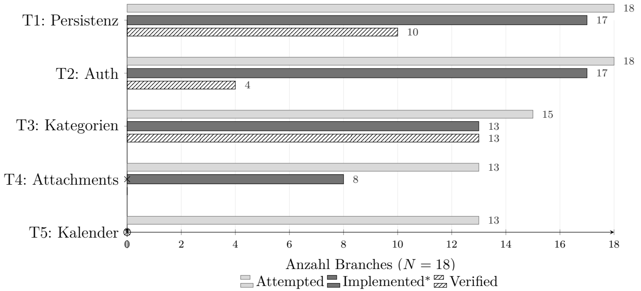
Abbildung 6.1: Pipeline-Ergebnisse für T1–T5 ( N = 18 ) als gruppierte Balken: Attempted (Chat-Signal), Implemented* (definiert als Attempted \wedge (Implemented_{static} \vee Verified) ) und Verified (testgebunden: bestandene V3-Integrationstests). Die Werte entsprechen Tabelle 6.2.
