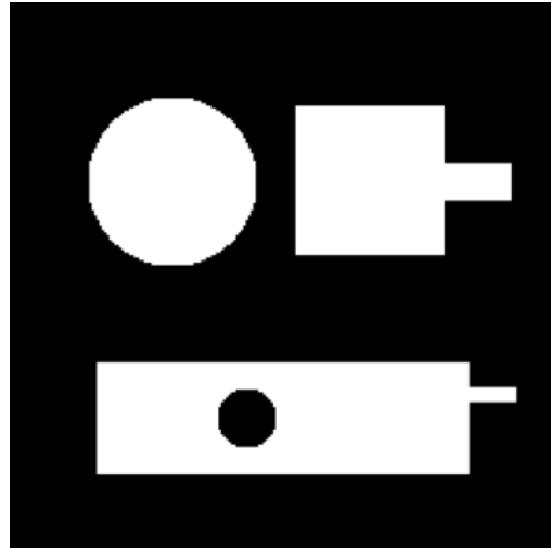
input set X
