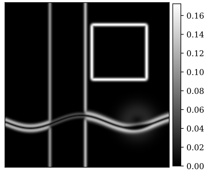
gradient magnitude
