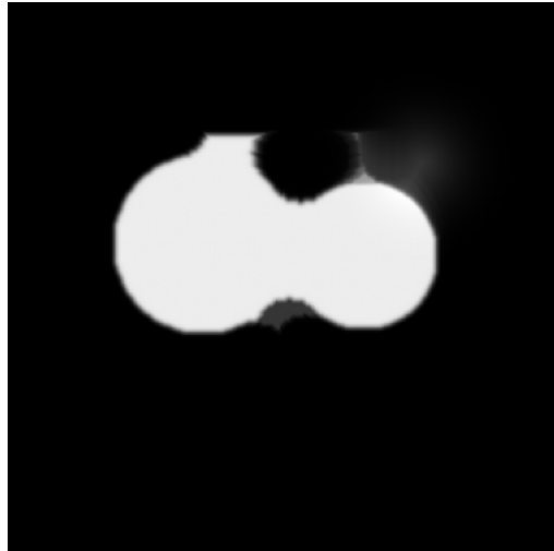
marker (erosion)
