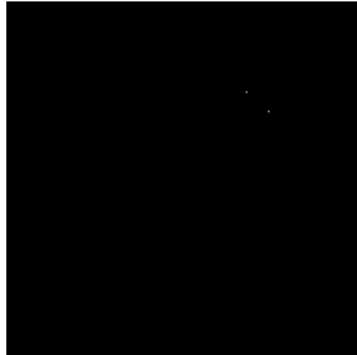
h -maxima
