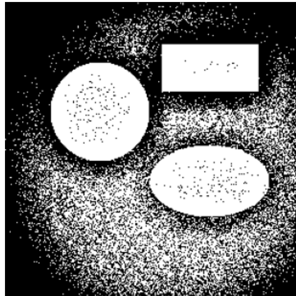
Sauvola Dice=0.647
