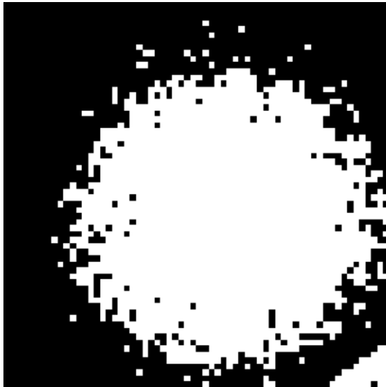
s-t min cut
