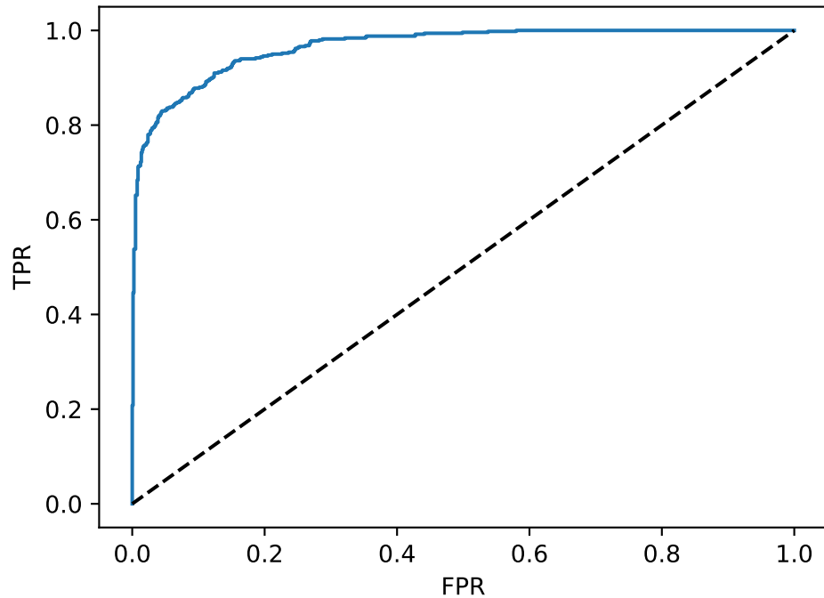
ROC, AUC = 0.966
