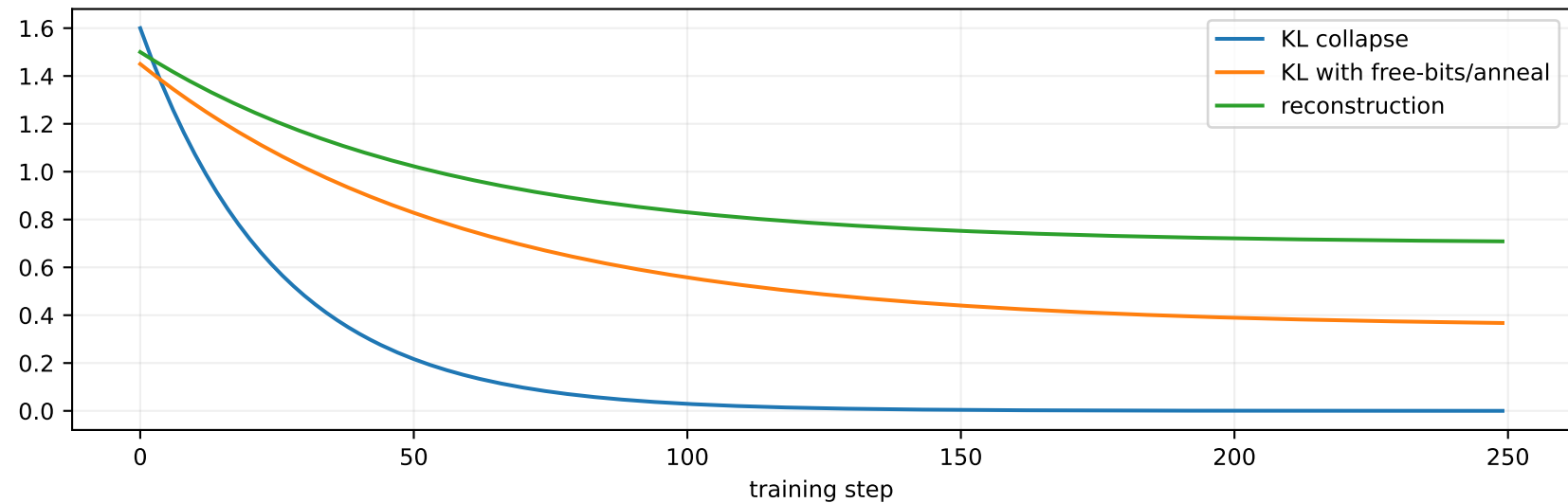
Posterior collapse diagnostics
