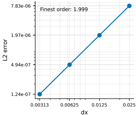
Diffusion only
