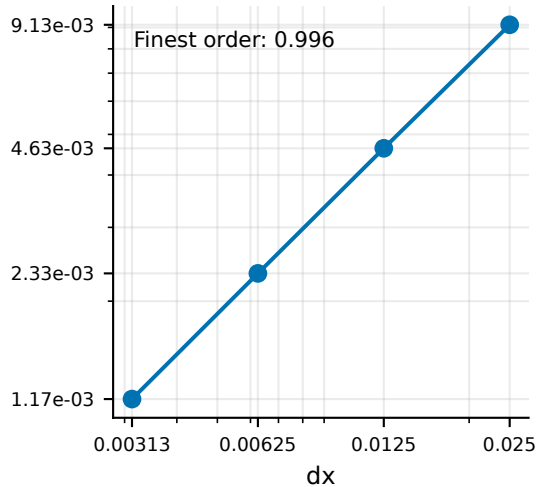
Upwind + diffusion
