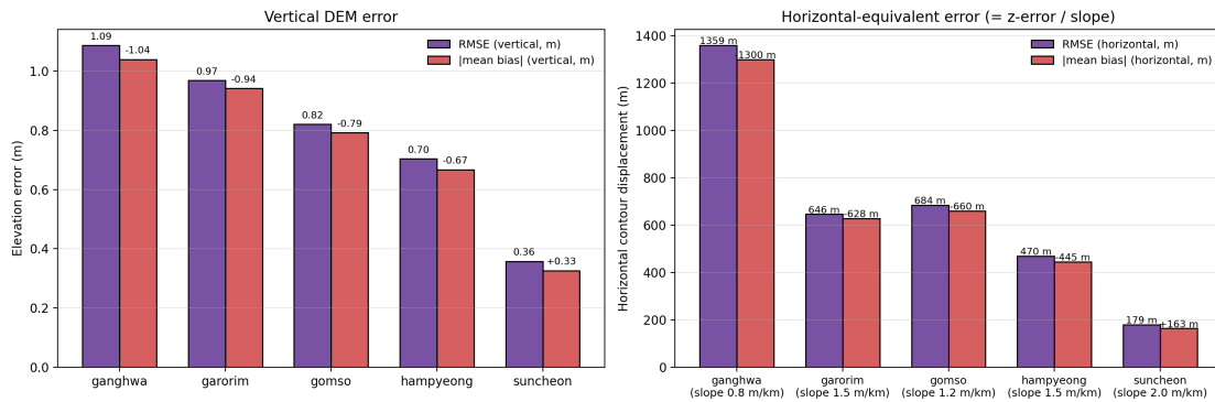
그림 7. 사이트별 워터라인-DEM 커버리지와 오차 예산. (a) 표본/누락 표고 띠: 회색 = 위성 표본 조위가 커버하는 표고 범위; 빨강 = 상부 절단 (회복 불능); 파랑 = 하부 절단. 절단 띠는 서해안에서 1.36–2.02 m, 순천만에서 0.99 m의 수직 범위를 차지하며 동일 통과 시각의 추가 광학 영상으로는 채울 수 없다. (b) 사이트별 수직 (좌)·수평 등가 (우) RMSE 및 |mean bias|의 세 센서 평균. 수평 RMSE는 수직 RMSE와 가정한 조건대 경사에 동시에 의존하며, 가장 완만한 강화도가 가장 큰 수평 오차 예산 (1.3 km 이상)을 갖는다.
