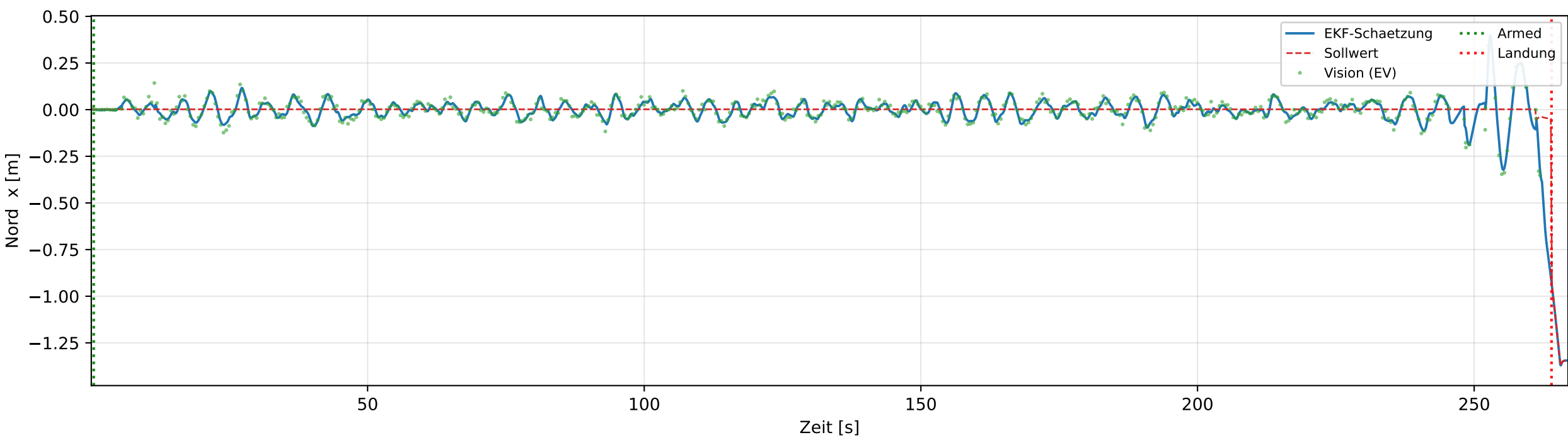
Position: Vision-Vorgabe vs. EKF-Schaetzung vs. Sollwert
