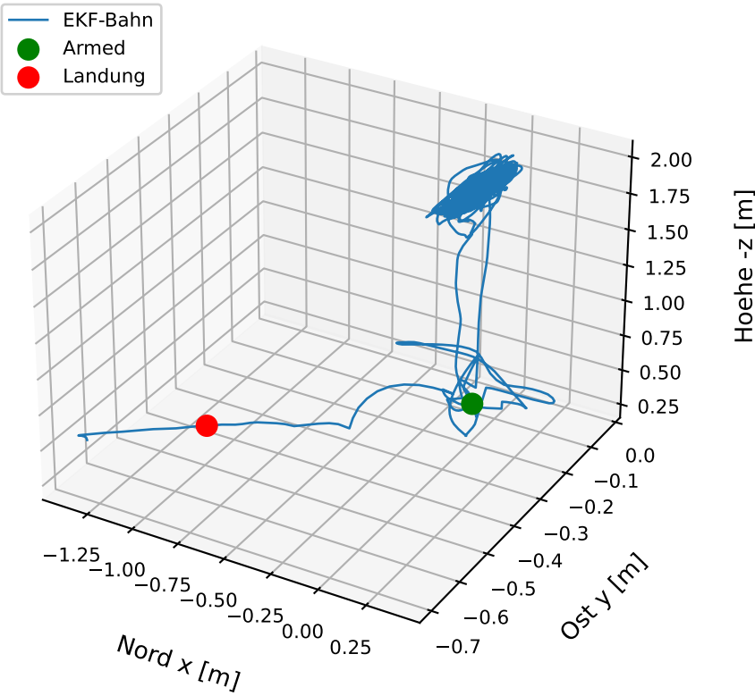
3D-Bahn
