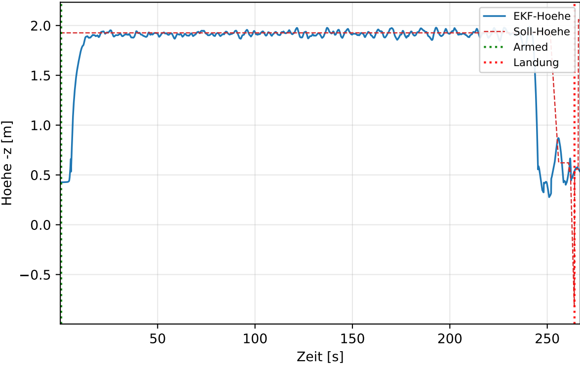
Hoehenverlauf
