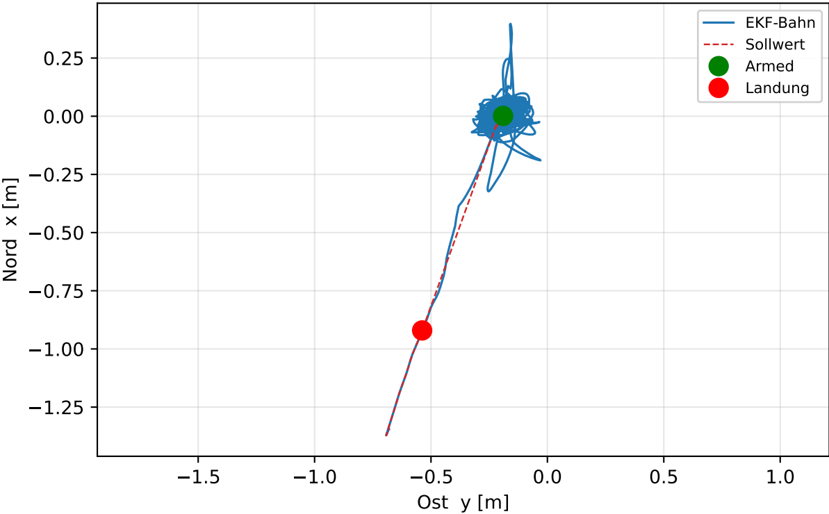
Draufsicht (XY)
