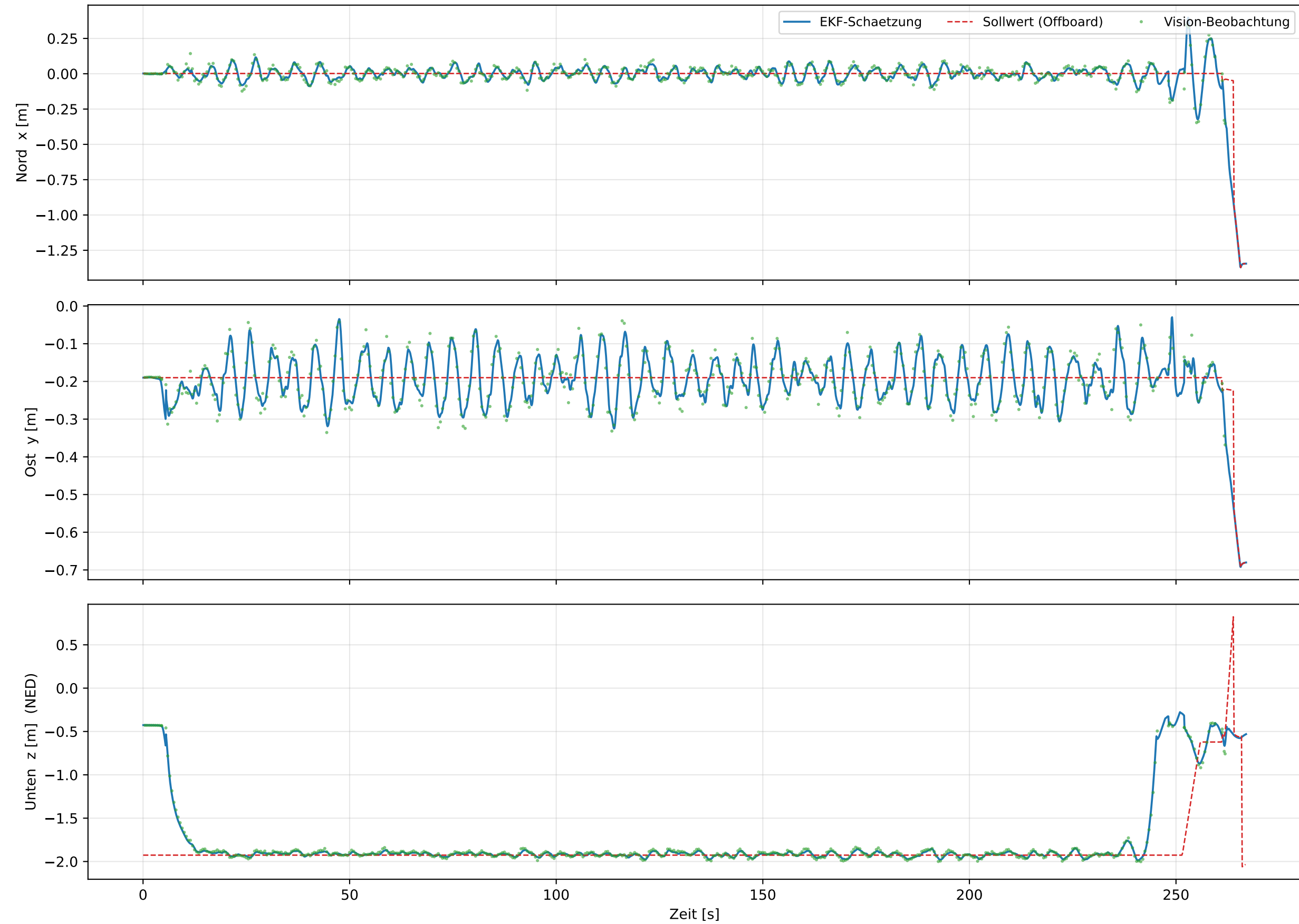
Position: Vision-Vorgabe vs. EKF-Schaetzung vs. Sollwert
