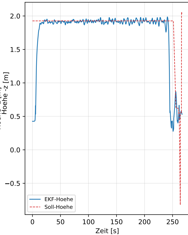
Hoehenverlauf
