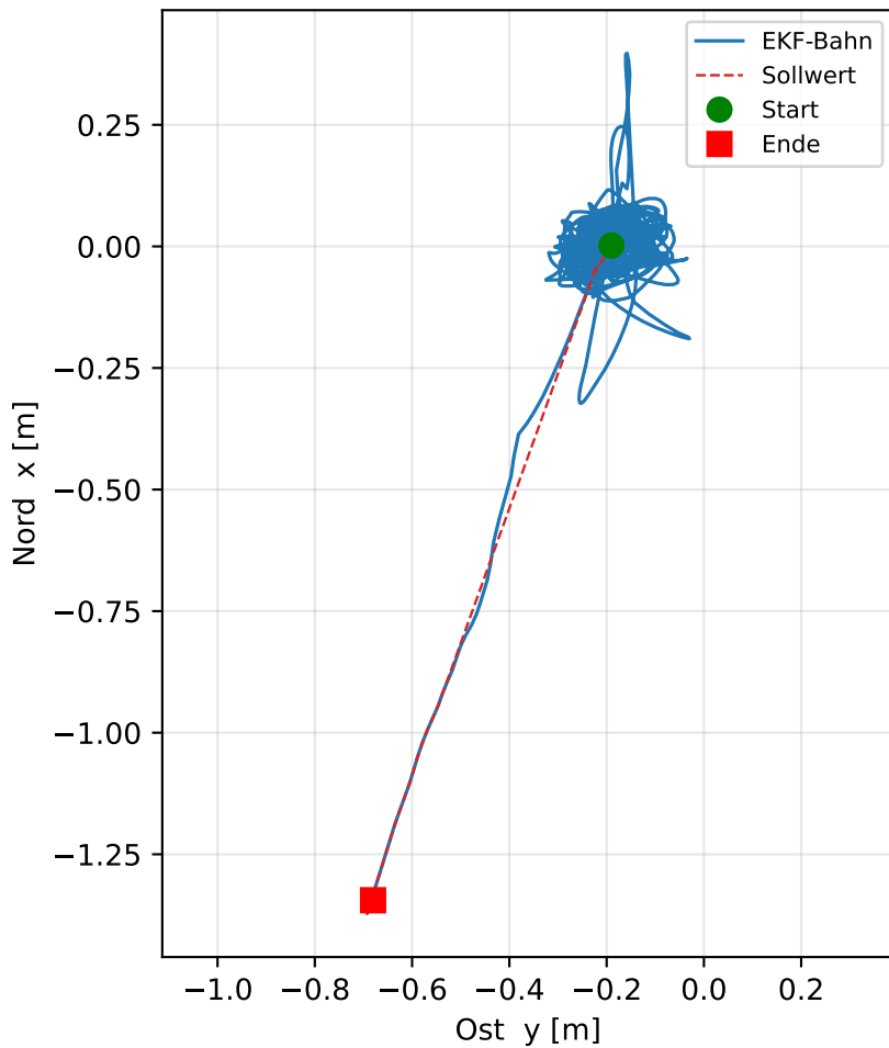
Draufsicht (XY)
