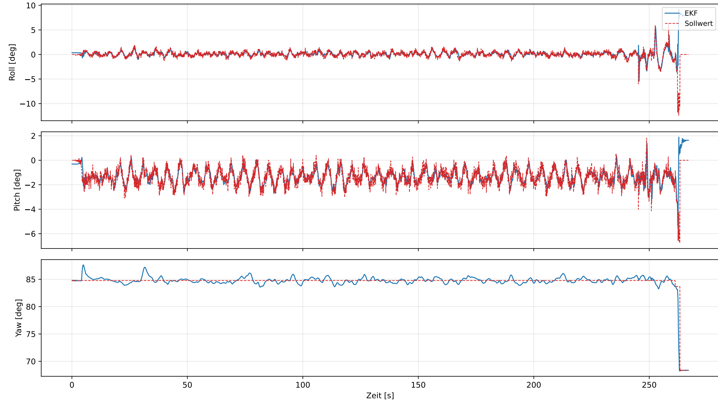
Lage: EKF vs. Sollwert
