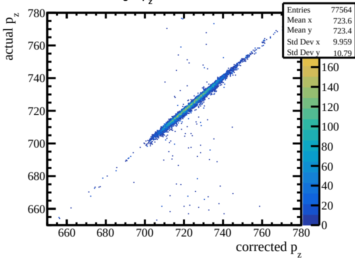
Target p_z : actual vs corrected
