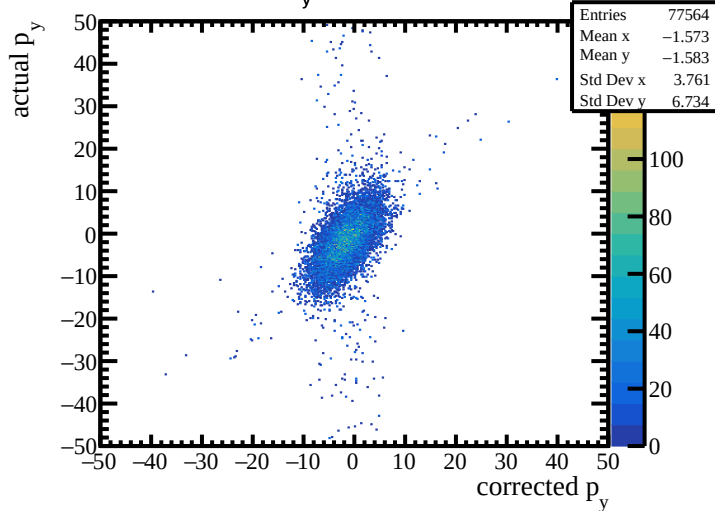
Target p_y : actual vs corrected
