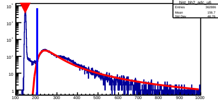
hist_bh2_adc_u6
