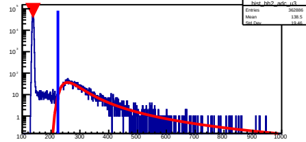
hist_bh2_adc_u3
