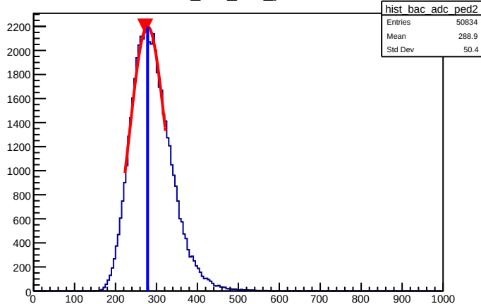
hist_bac_adc_ped2
