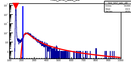
hist_bh2_adc_d8
