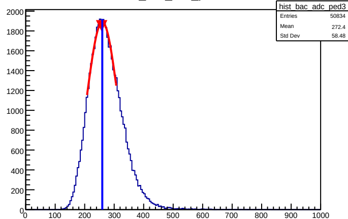
hist_bac_adc_ped3
