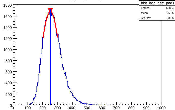
hist_bac_adc_ped1
