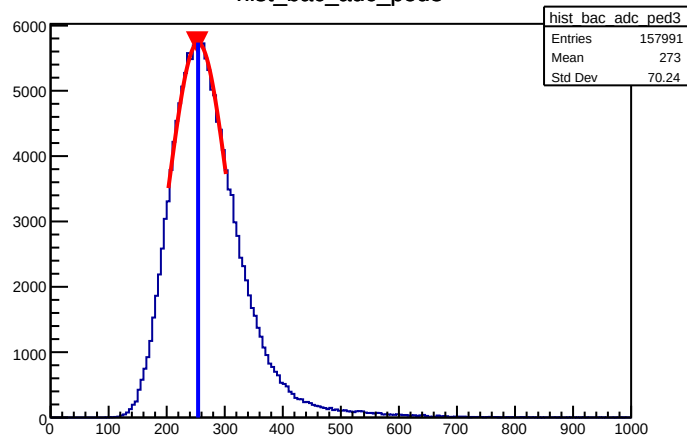
hist_bac_adc_ped3
