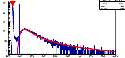
hist_bh2_adc_d4
