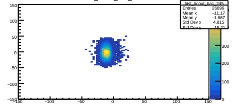
hist_bcout_bac_2d5
