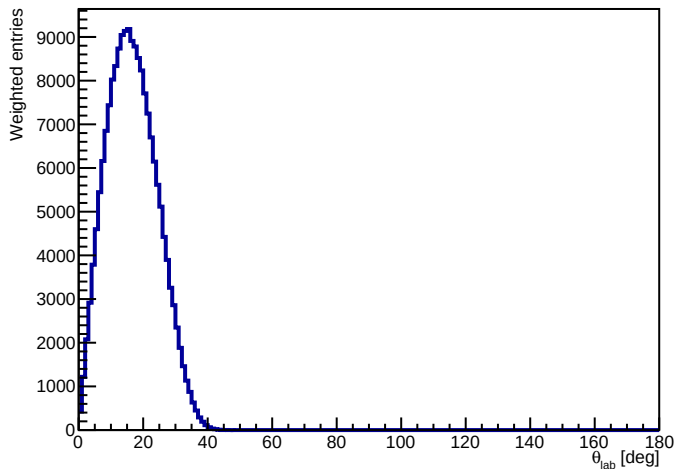
proton_all
