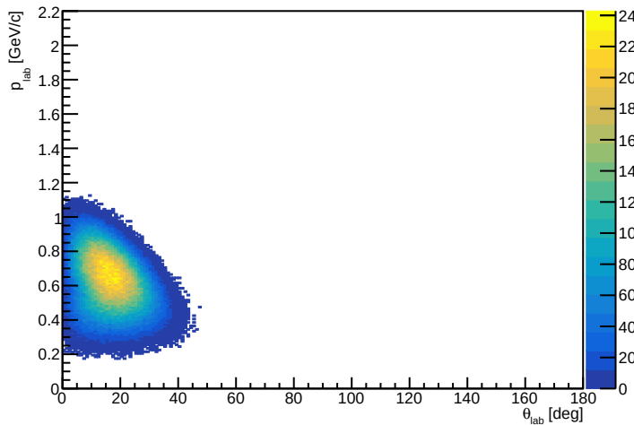
proton_all
