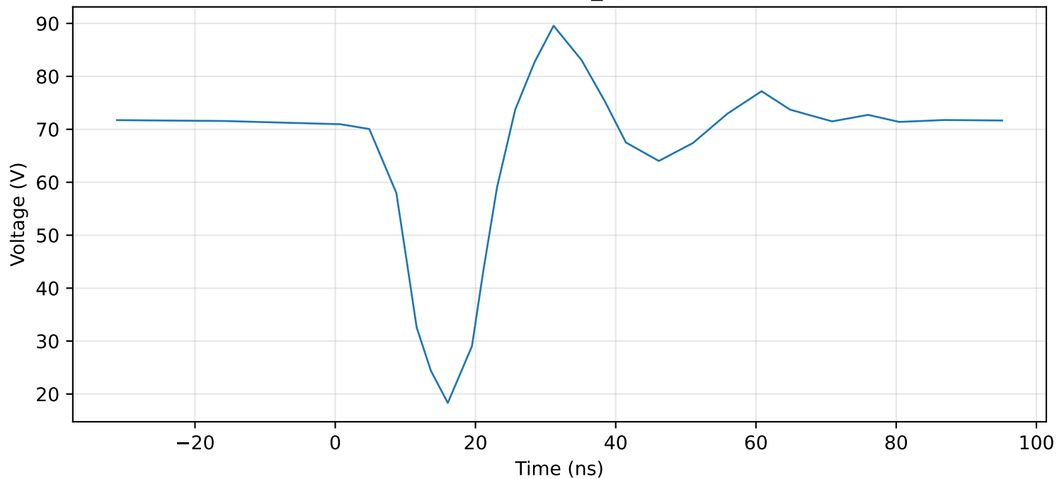
Waveform: rf_1k.csv
