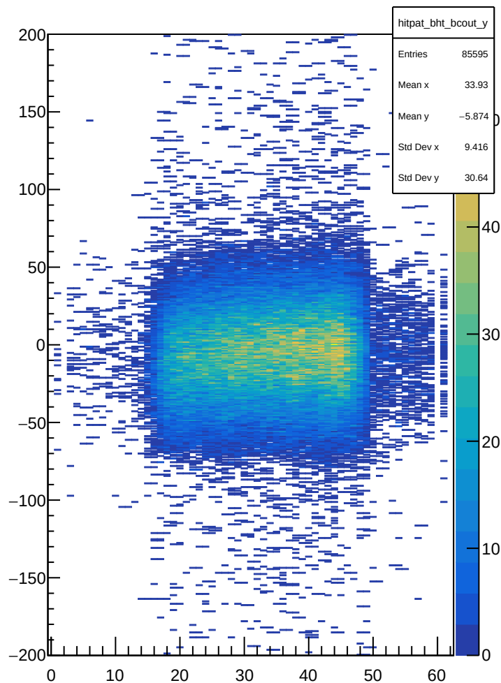
hitpat_bht_bcout_y
