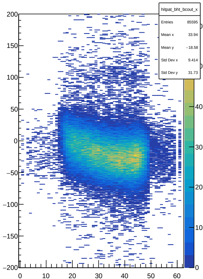
hitpat_bht_bcout_x
