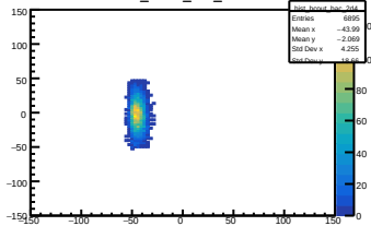
hist_bcout_bac_2d4
