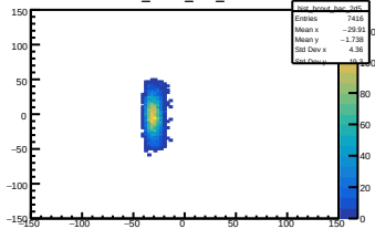
hist_bcout_bac_2d5
