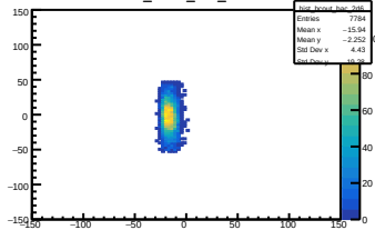
hist_bcout_bac_2d6
