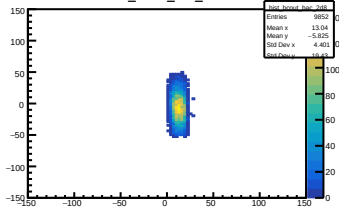
hist_bcout_bac_2d8
