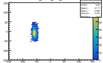
hist_bcout_bac_2d3
