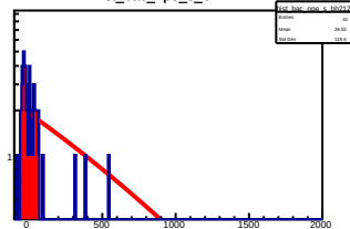
hist_bac_npe_s_bh212
