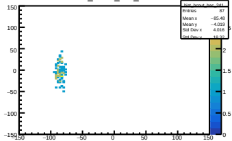
hist_bcout_bac_2d1
