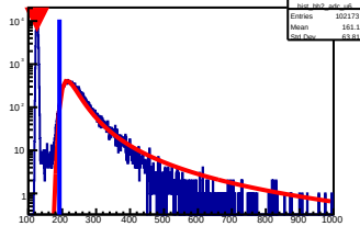
hist_bh2_adc_u6
