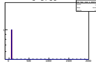
hist_bac_npe_s_bh213
