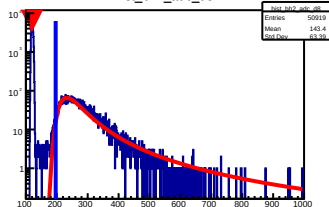
hist_bh2_adc_d8
