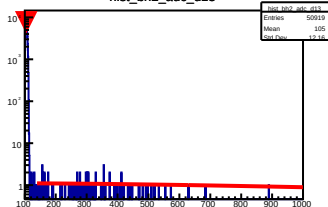
hist_bh2_adc_d13
