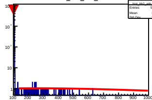
hist_bh2_adc_u2
