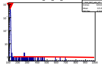
hist_bh2_adc_d2
