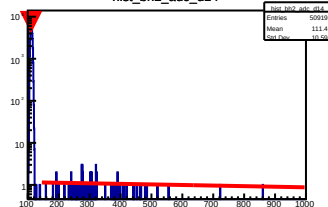
hist_bh2_adc_d14
