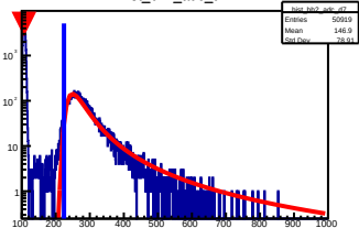
hist_bh2_adc_d7
