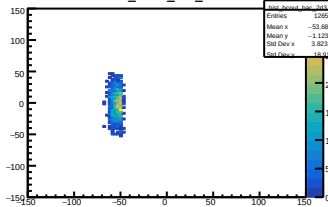
hist_bcout_bac_2d3
