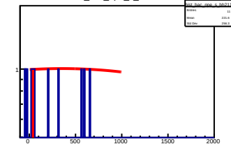
hist_bac_npe_s_bh211
