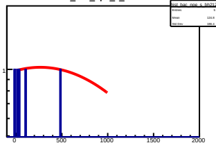
hist_bac_npe_s_bh212
