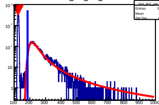
hist_bh2_adc_u6
