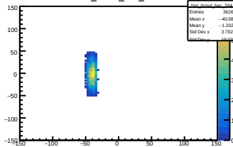
hist_bcout_bac_2d4
