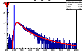
hist_bh2_adc_d6
