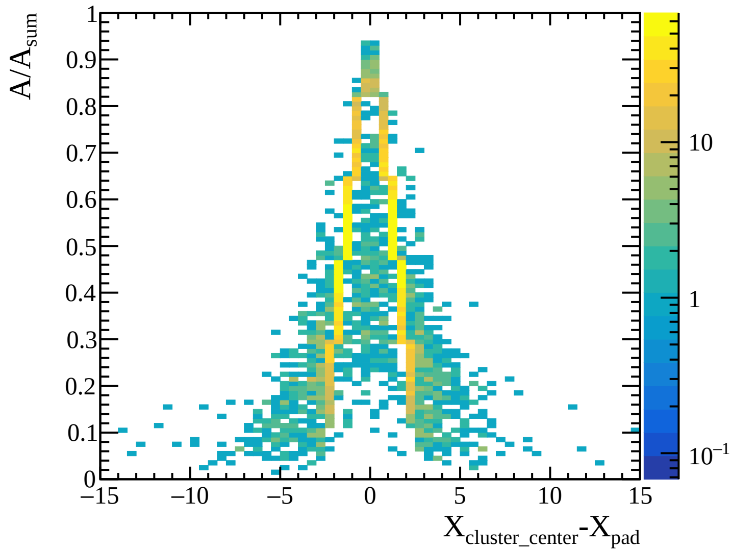
TPC transverse diffusion: layer 17 [Transverse_Diffusion_Layer17]
