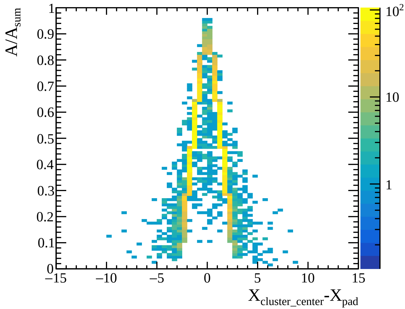
TPC transverse diffusion: layer 27 [Transverse_Diffusion_Layer27]
