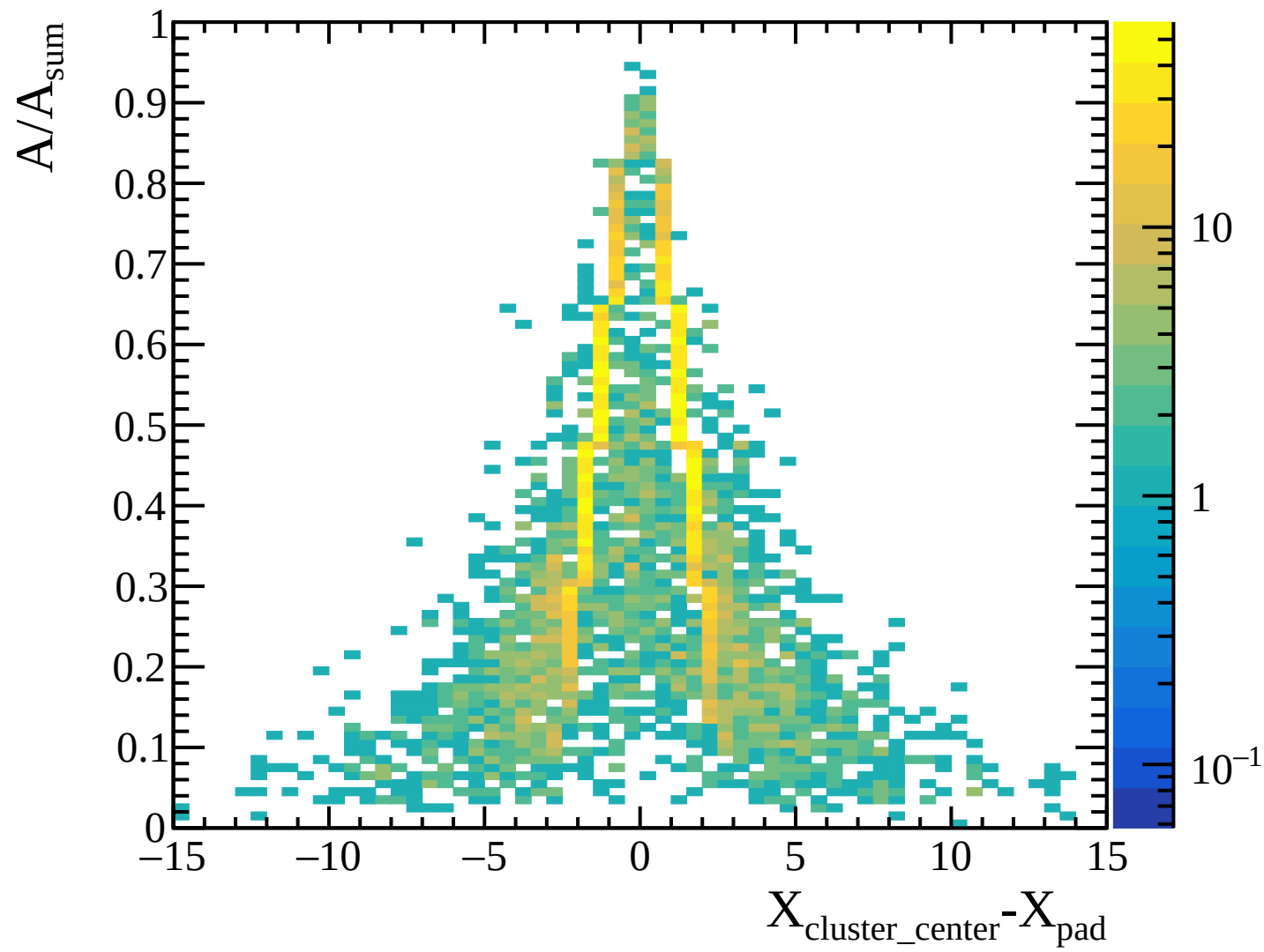
TPC transverse diffusion: layer 13 [Transverse_Diffusion_Layer13]
