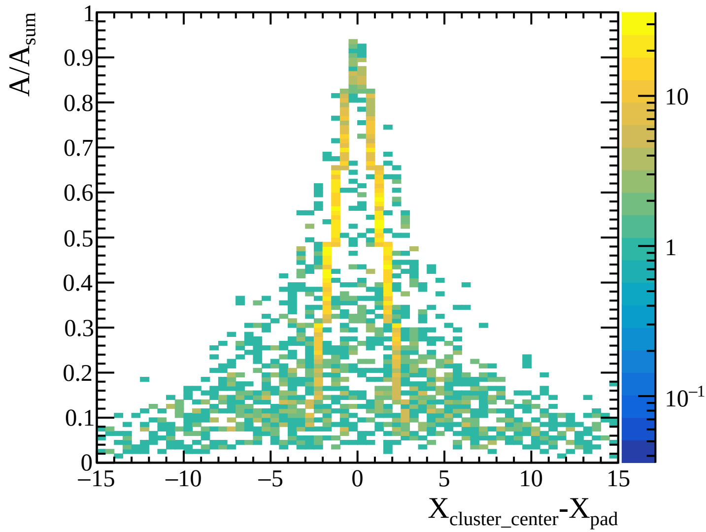
TPC transverse diffusion: layer 10 [Transverse_Diffusion_Layer10]
