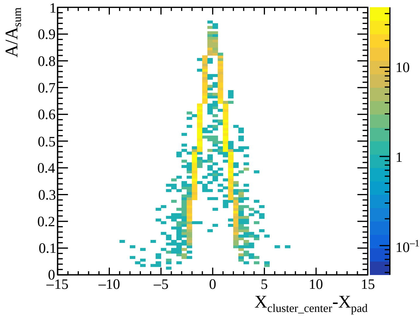
TPC transverse diffusion: layer 31 [Transverse_Diffusion_Layer31]
