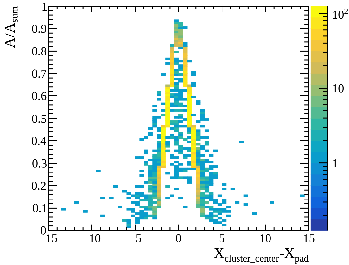
TPC transverse diffusion: layer 29 [Transverse_Diffusion_Layer29]
