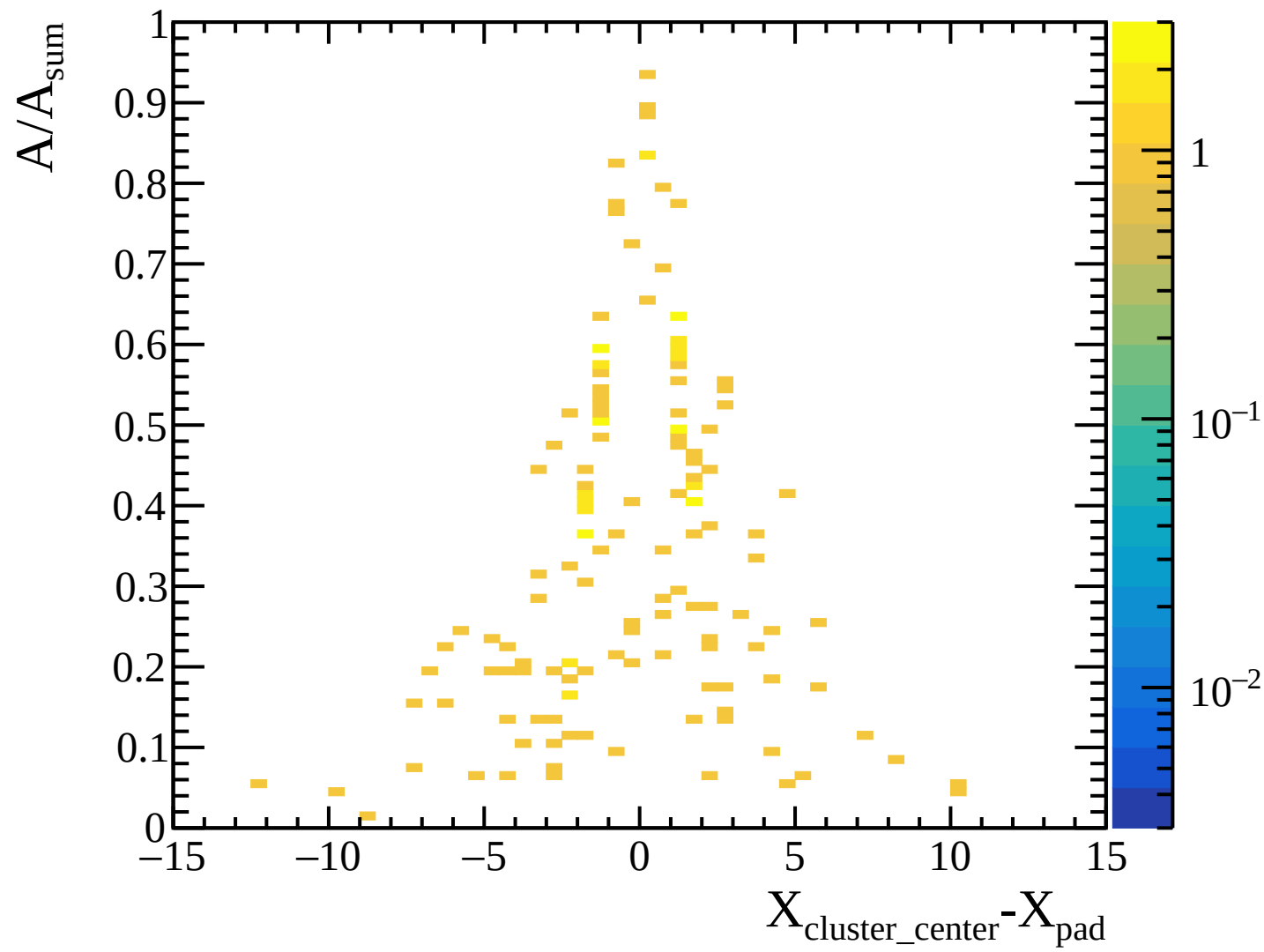
TPC transverse diffusion: layer 03 [Transverse_Diffusion_Layer03]
