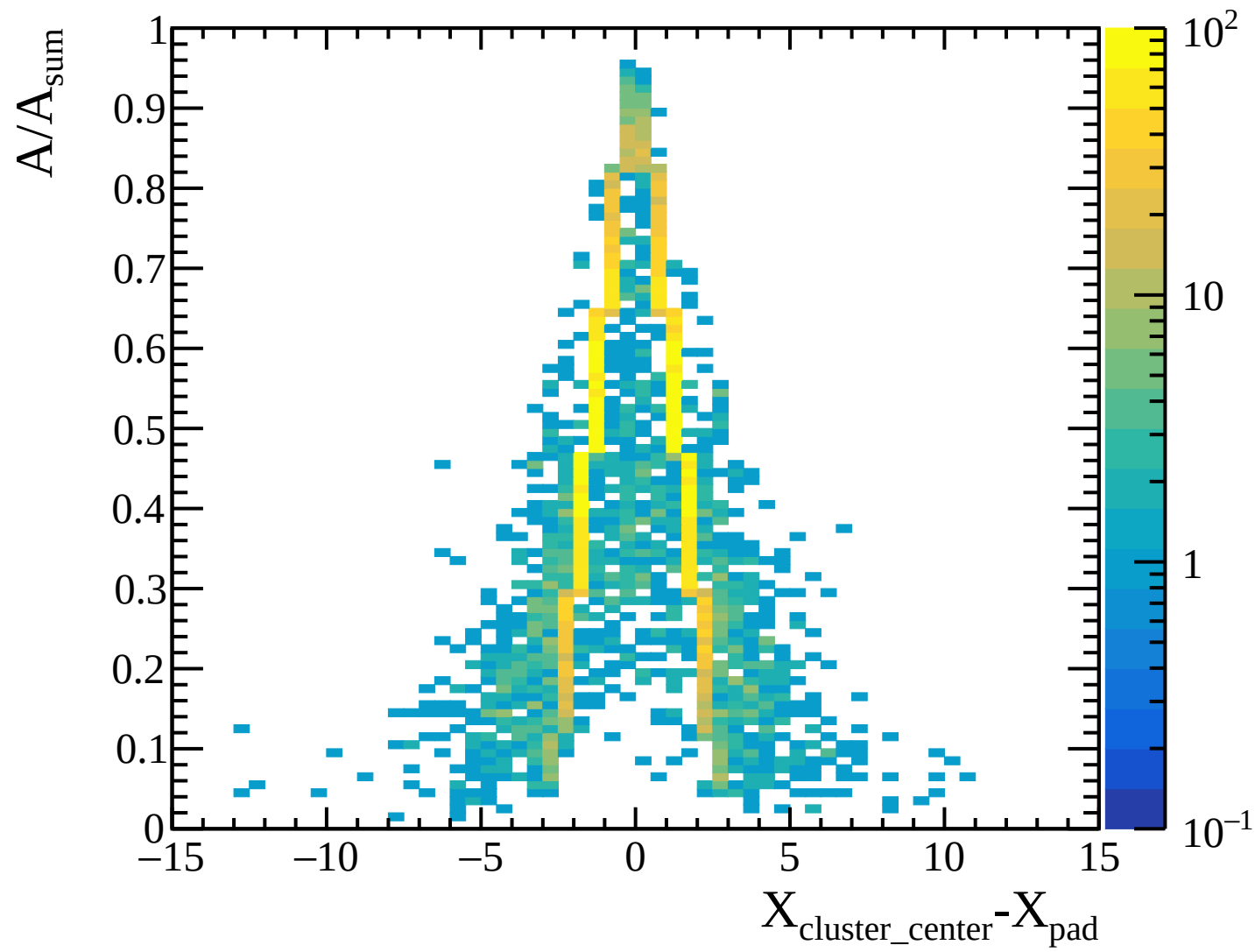
TPC transverse diffusion: layer 18 [Transverse_Diffusion_Layer18]
