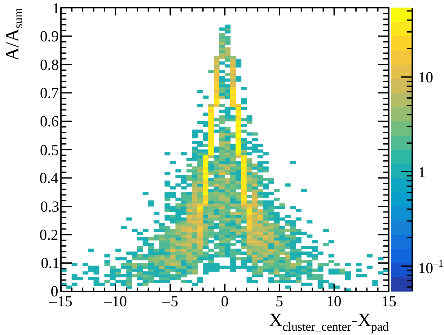
TPC transverse diffusion: layer 12 [Transverse_Diffusion_Layer12]
