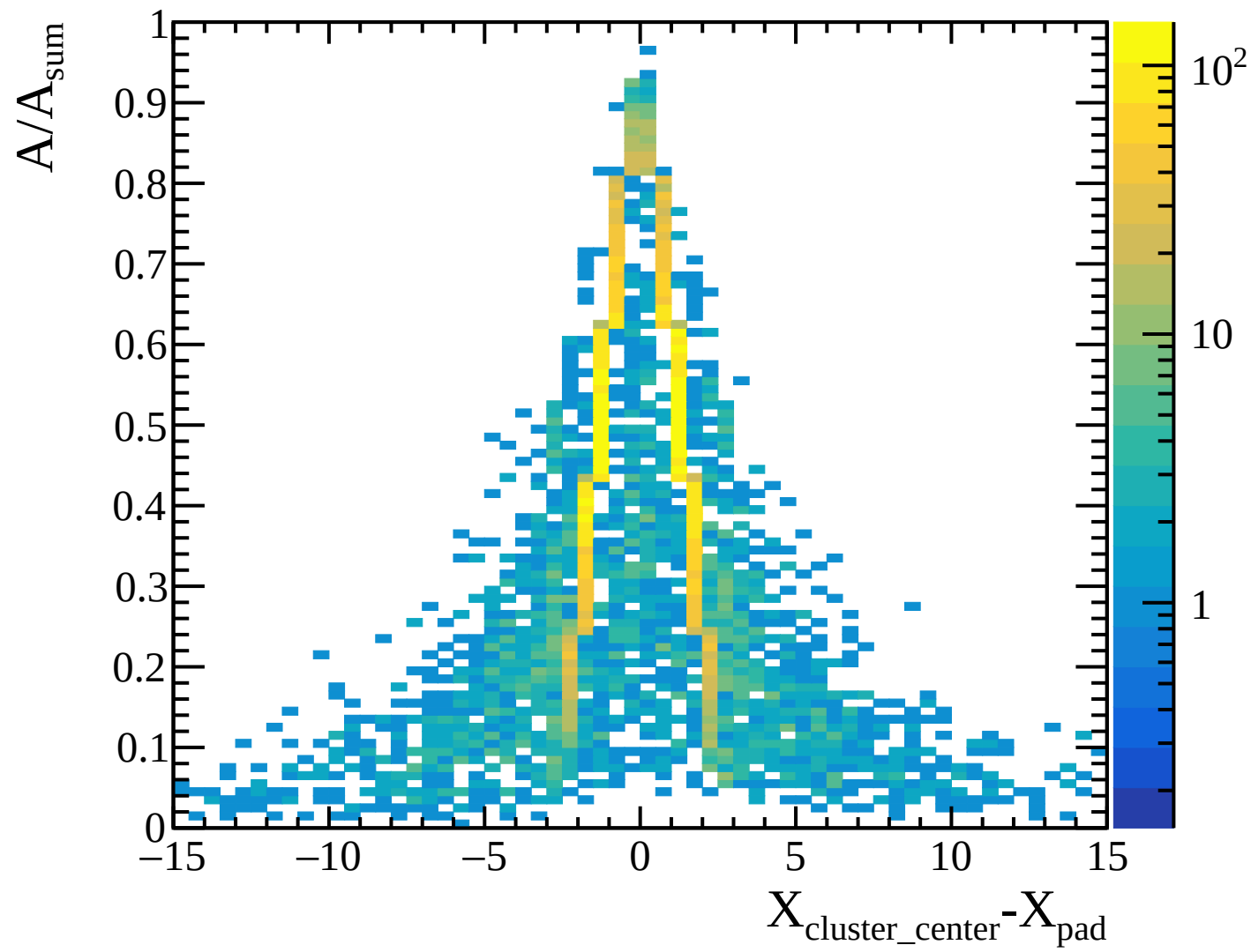
TPC transverse diffusion: layer 08 [Transverse_Diffusion_Layer08]
