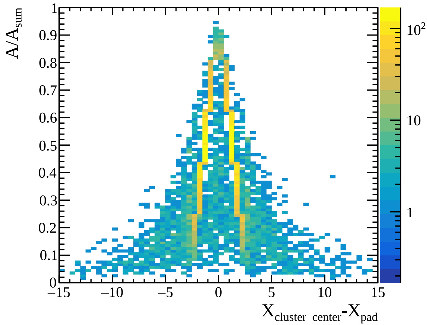
TPC transverse diffusion: layer 07 [Transverse_Diffusion_Layer07]
