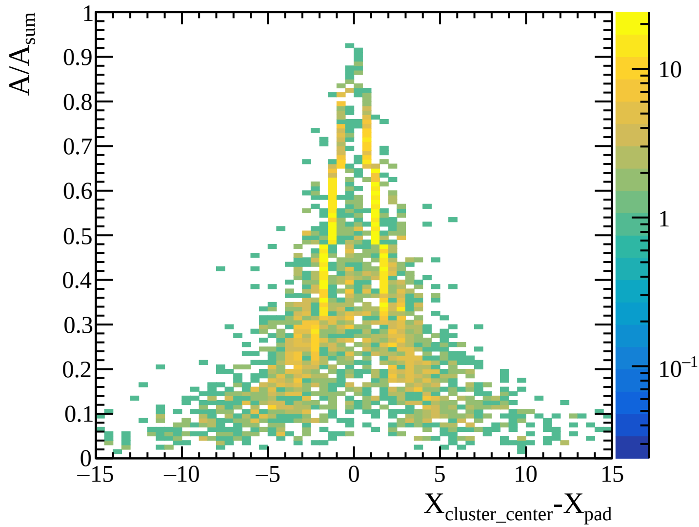
TPC transverse diffusion: layer 11 [Transverse_Diffusion_Layer11]
