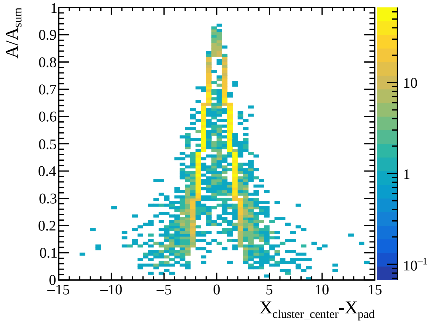
TPC transverse diffusion: layer 16 [Transverse_Diffusion_Layer16]
