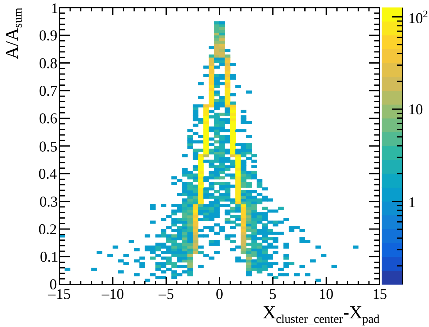
TPC transverse diffusion: layer 20 [Transverse_Diffusion_Layer20]
