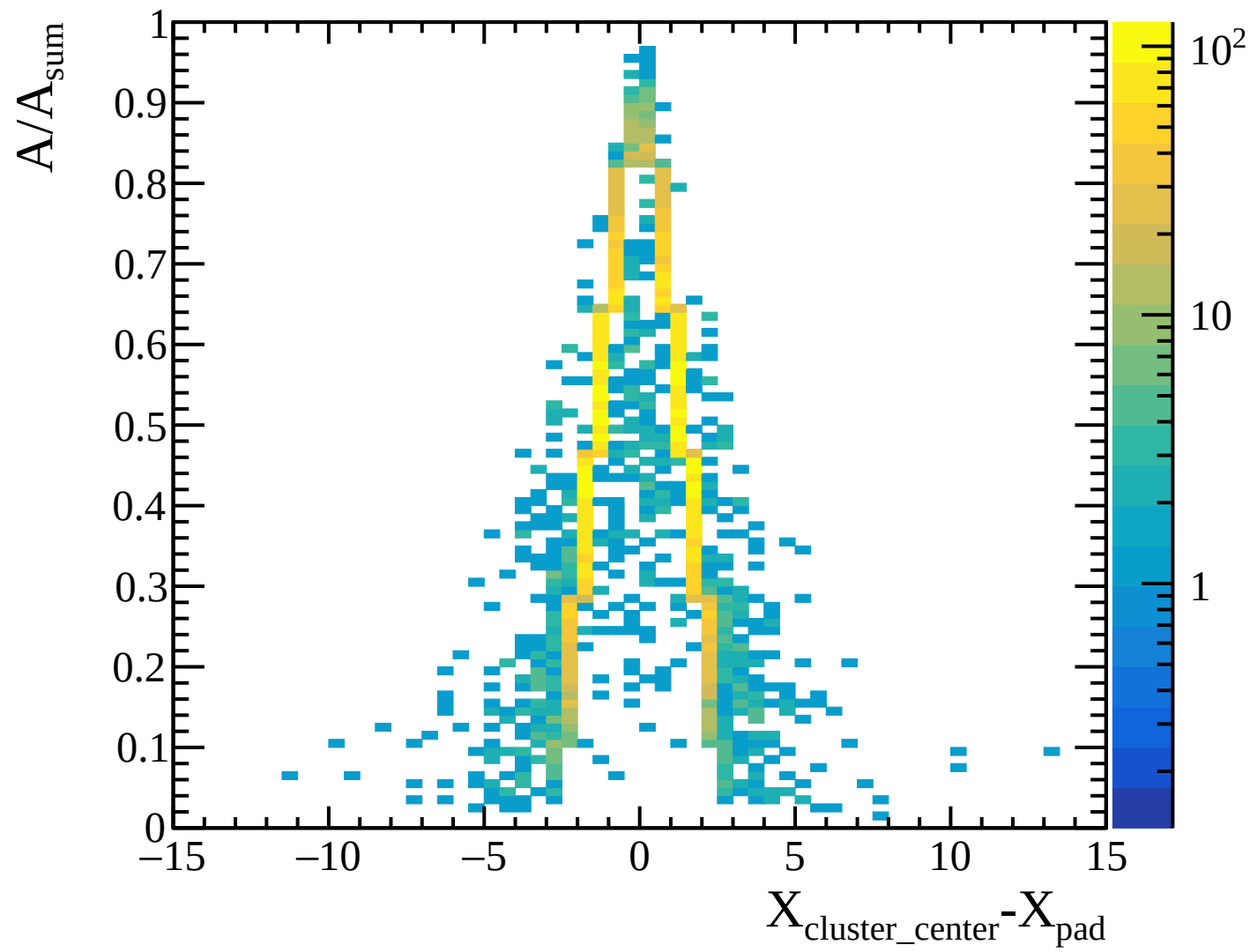
TPC transverse diffusion: layer 26 [Transverse_Diffusion_Layer26]
