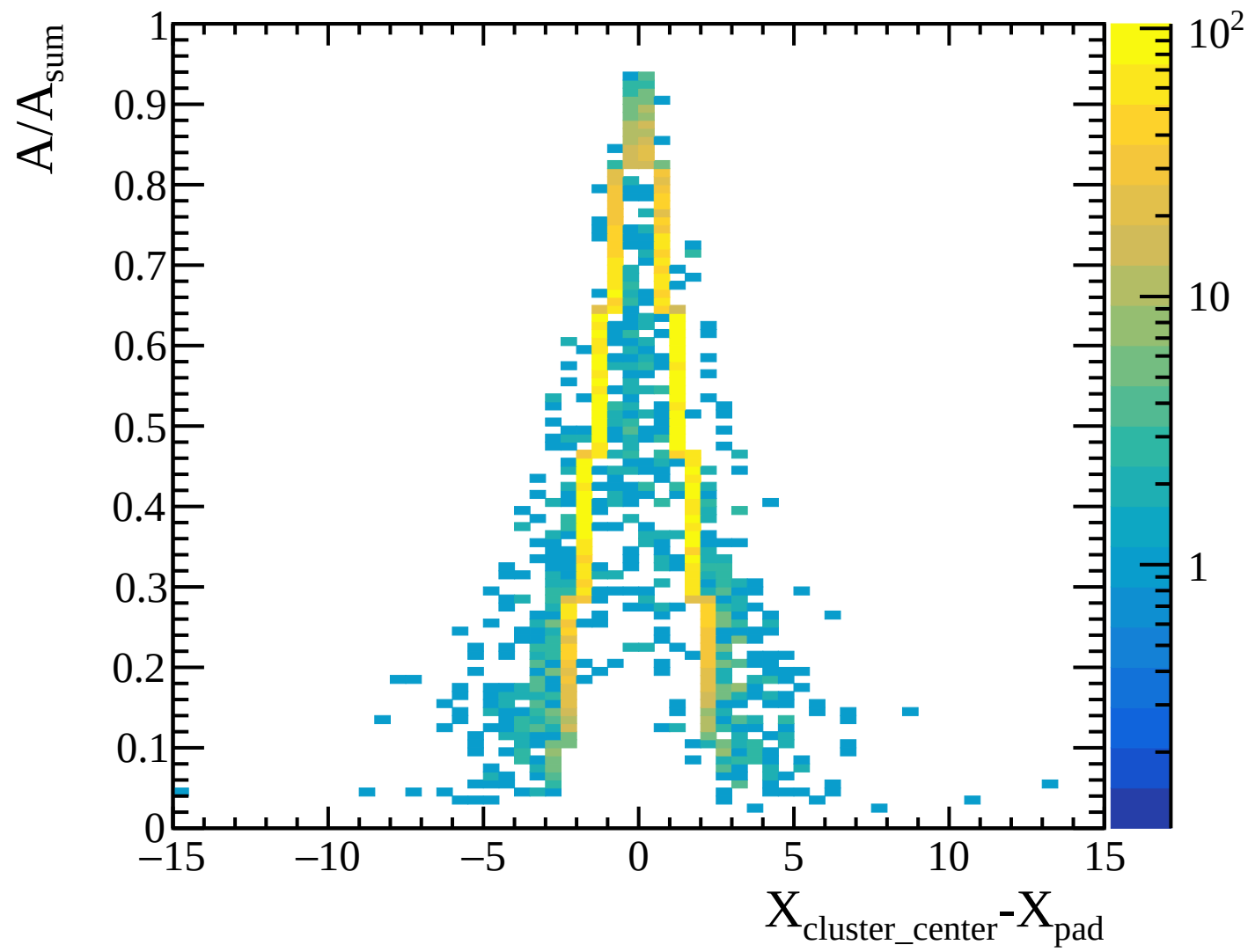
TPC transverse diffusion: layer 25 [Transverse_Diffusion_Layer25]
