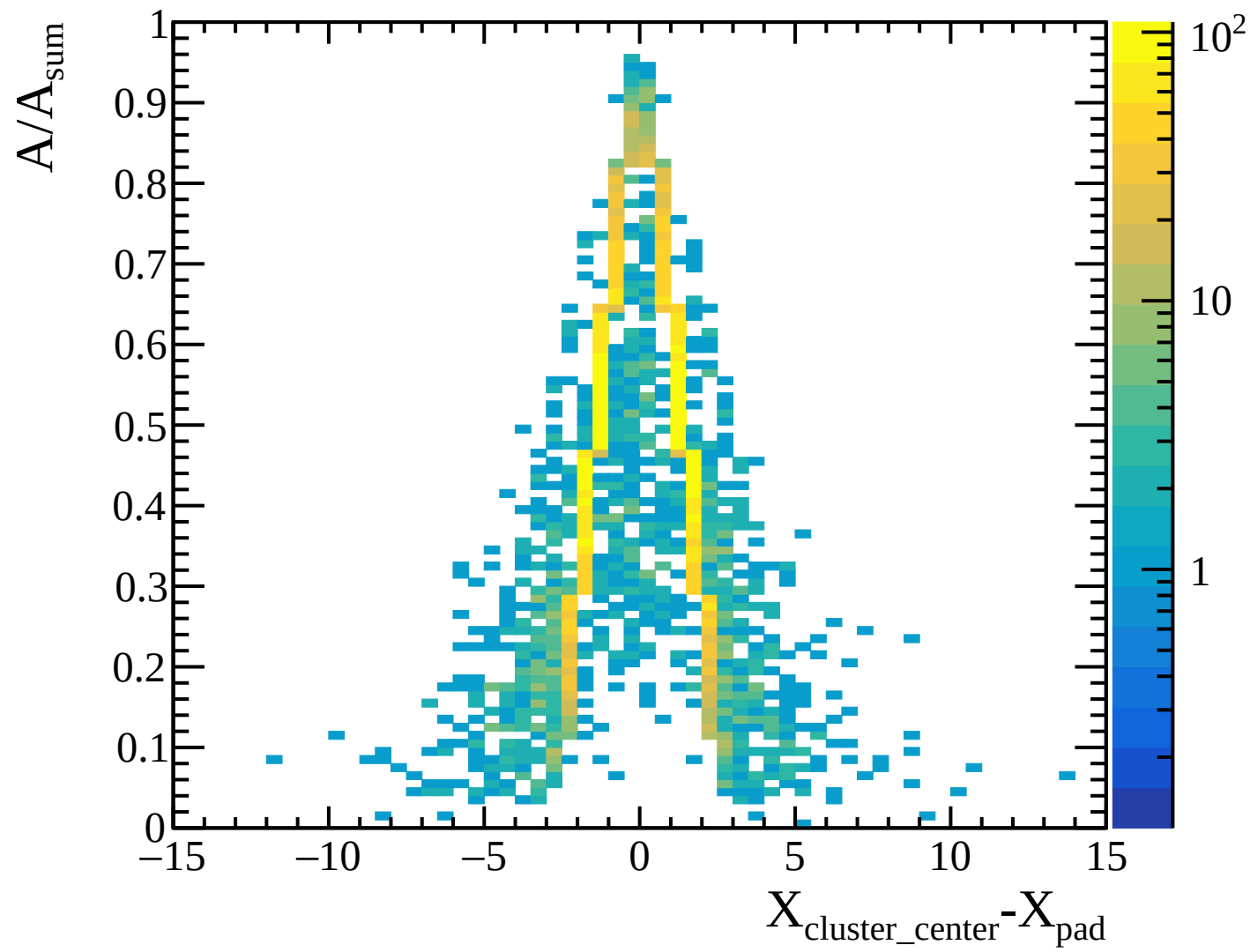
TPC transverse diffusion: layer 19 [Transverse_Diffusion_Layer19]
