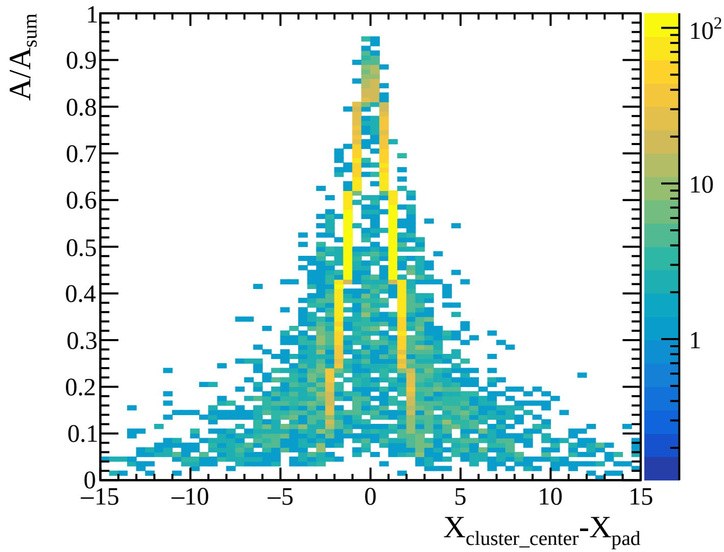
TPC transverse diffusion: layer 09 [Transverse_Diffusion_Layer09]
