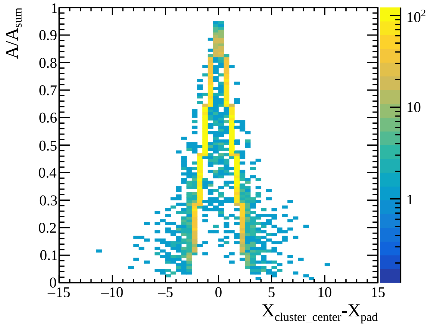
TPC transverse diffusion: layer 24 [Transverse_Diffusion_Layer24]
