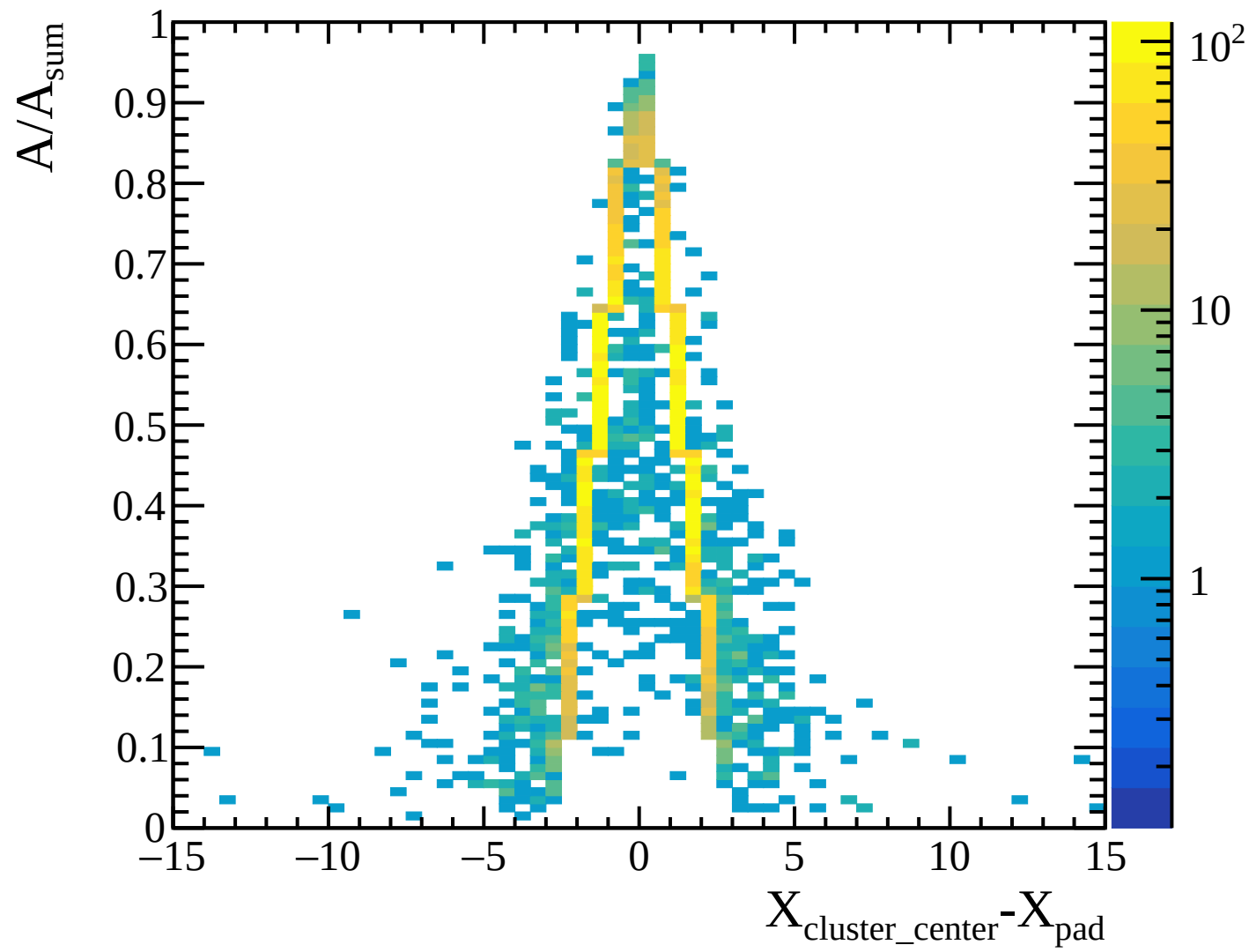
TPC transverse diffusion: layer 23 [Transverse_Diffusion_Layer23]
