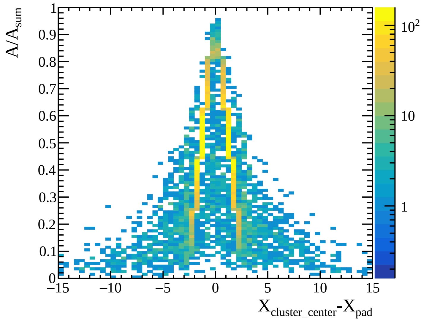
TPC transverse diffusion: layer 06 [Transverse_Diffusion_Layer06]
