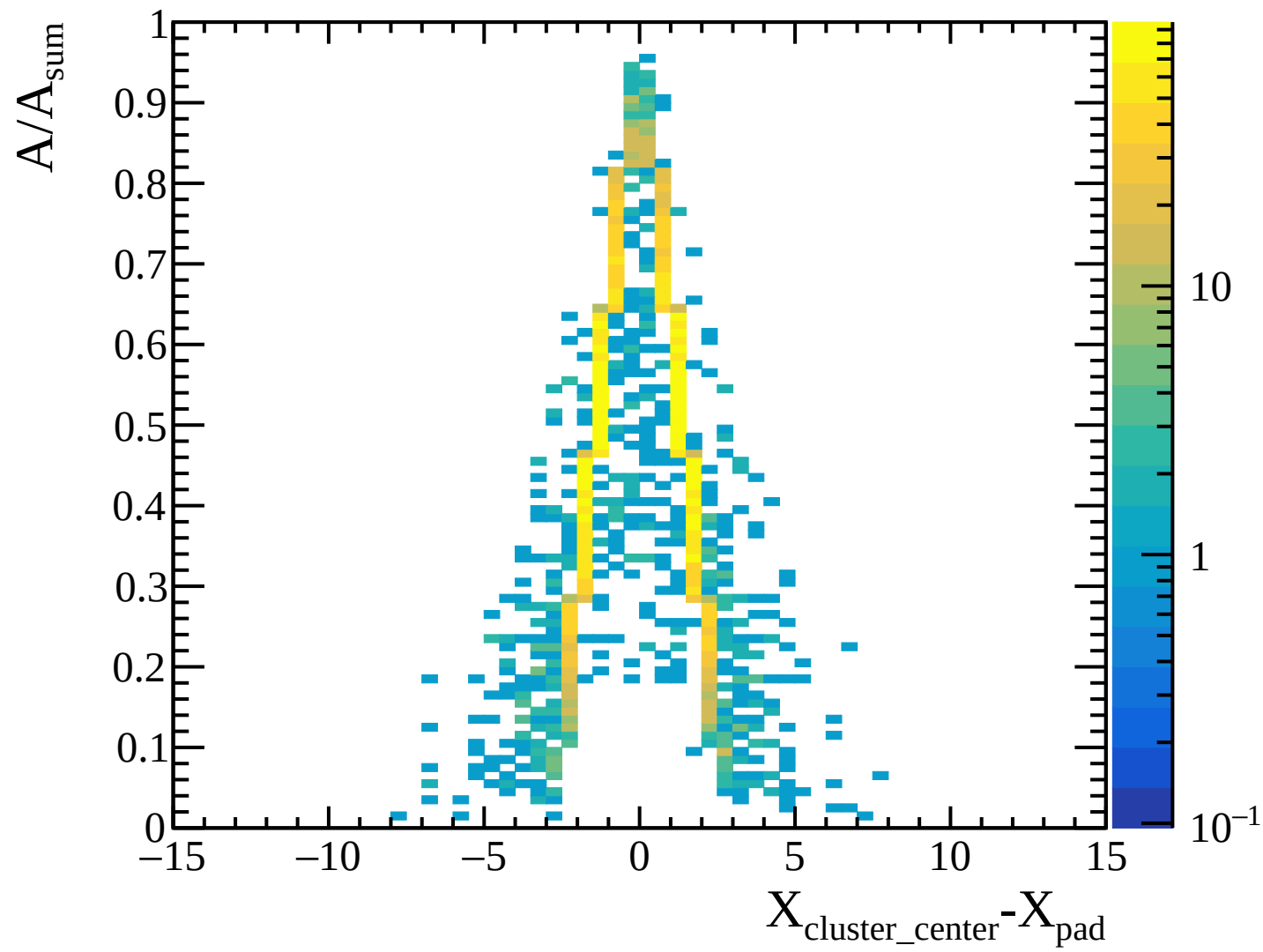
TPC transverse diffusion: layer 30 [Transverse_Diffusion_Layer30]
