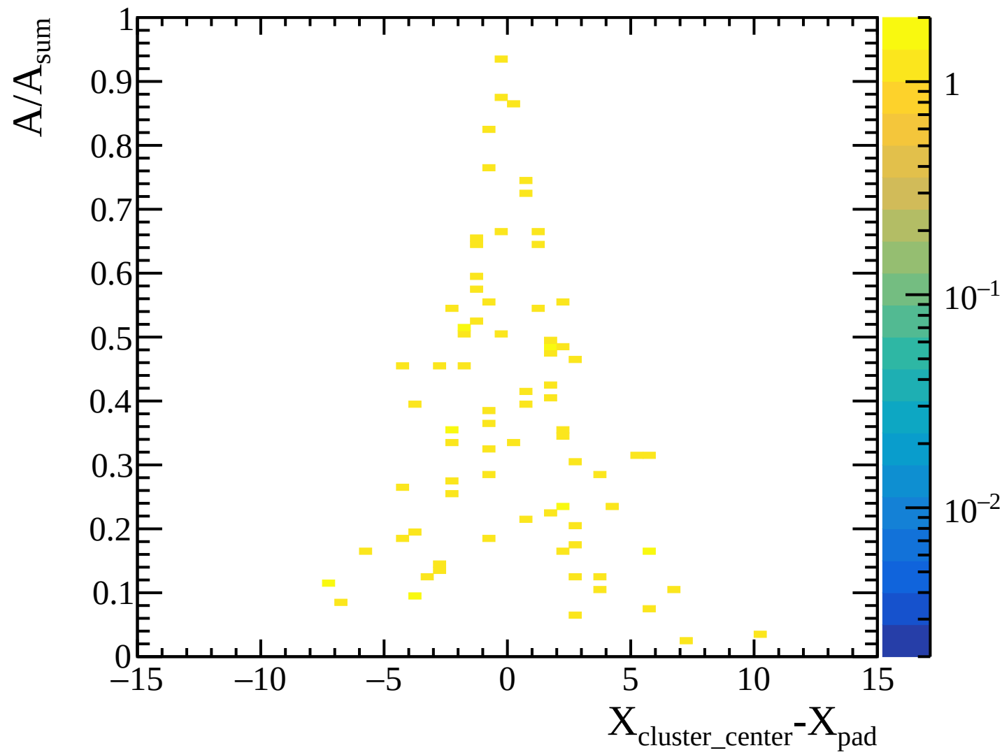
TPC transverse diffusion: layer 01 [Transverse_Diffusion_Layer01]
