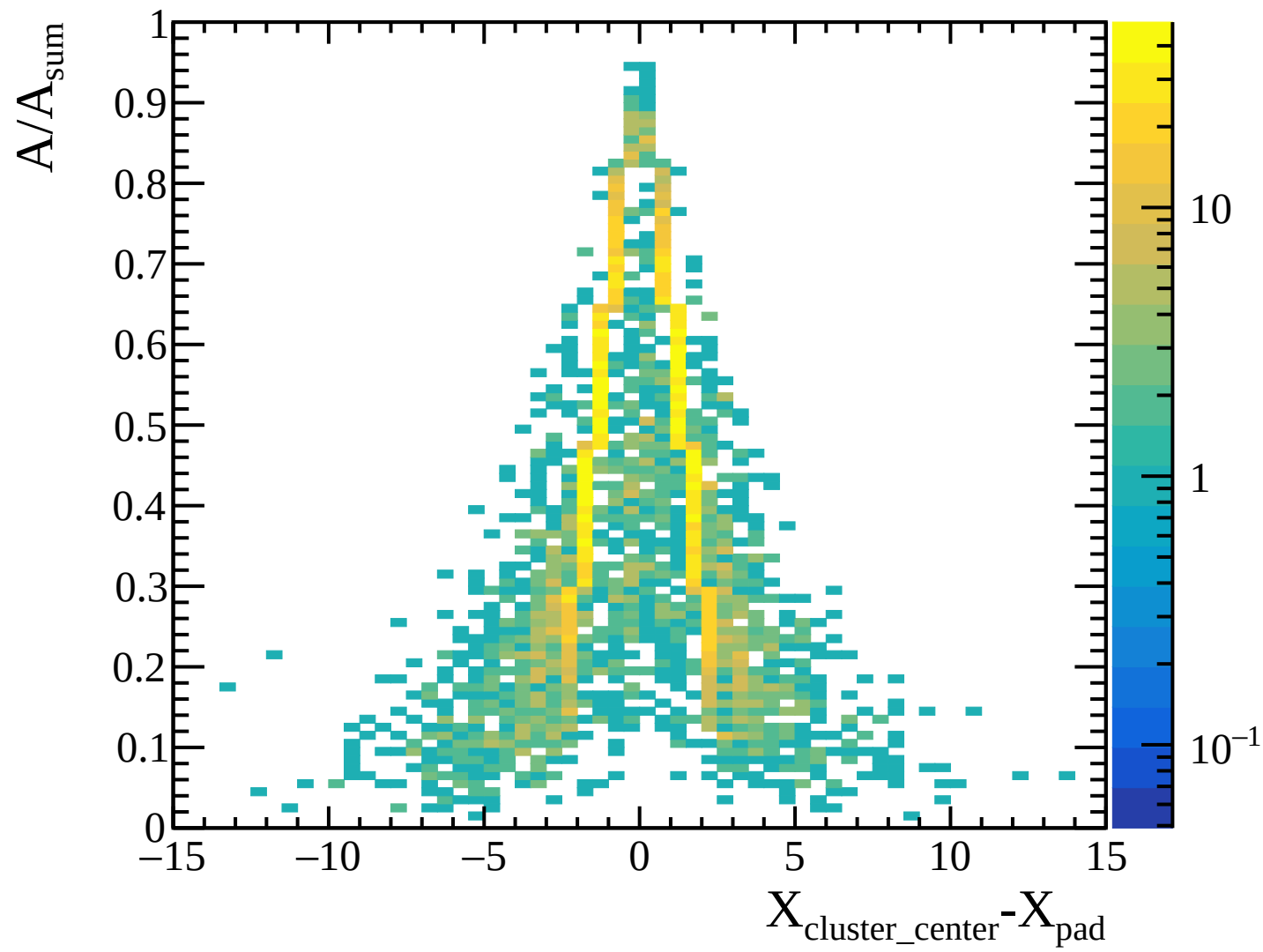
TPC transverse diffusion: layer 15 [Transverse_Diffusion_Layer15]
