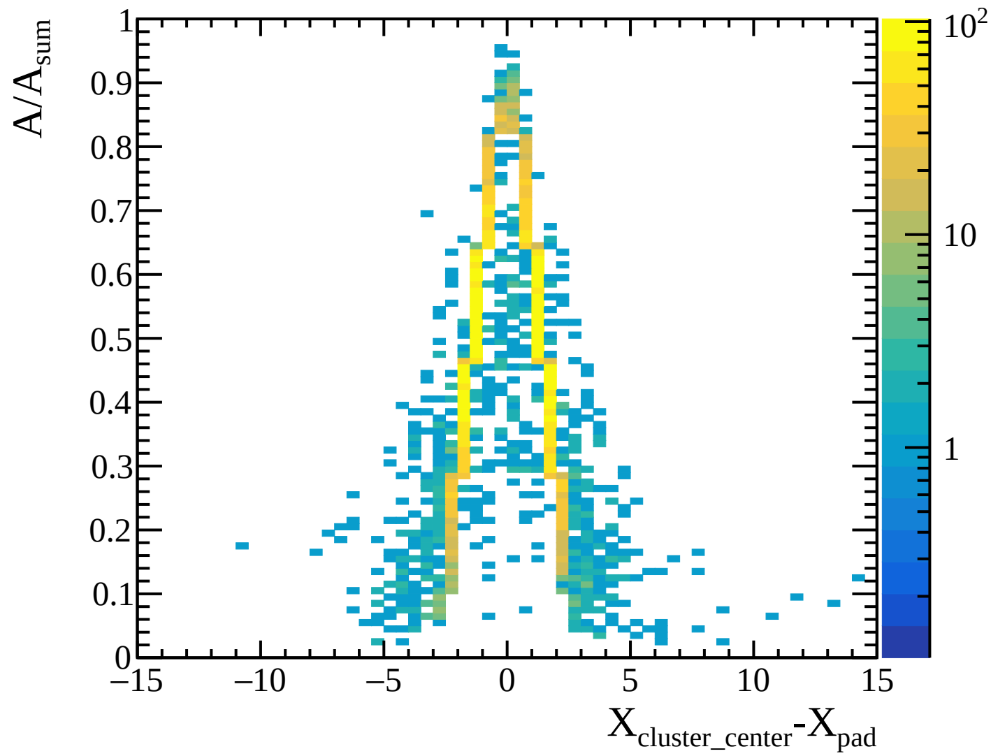
TPC transverse diffusion: layer 28 [Transverse_Diffusion_Layer28]
