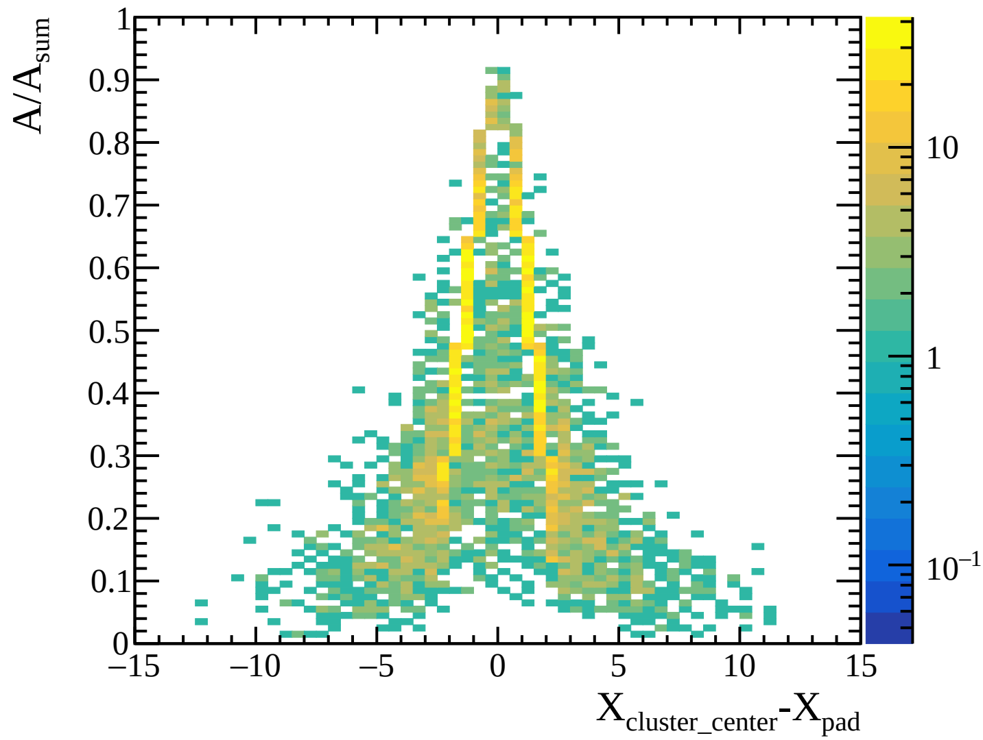
TPC transverse diffusion: layer 14 [Transverse_Diffusion_Layer14]
