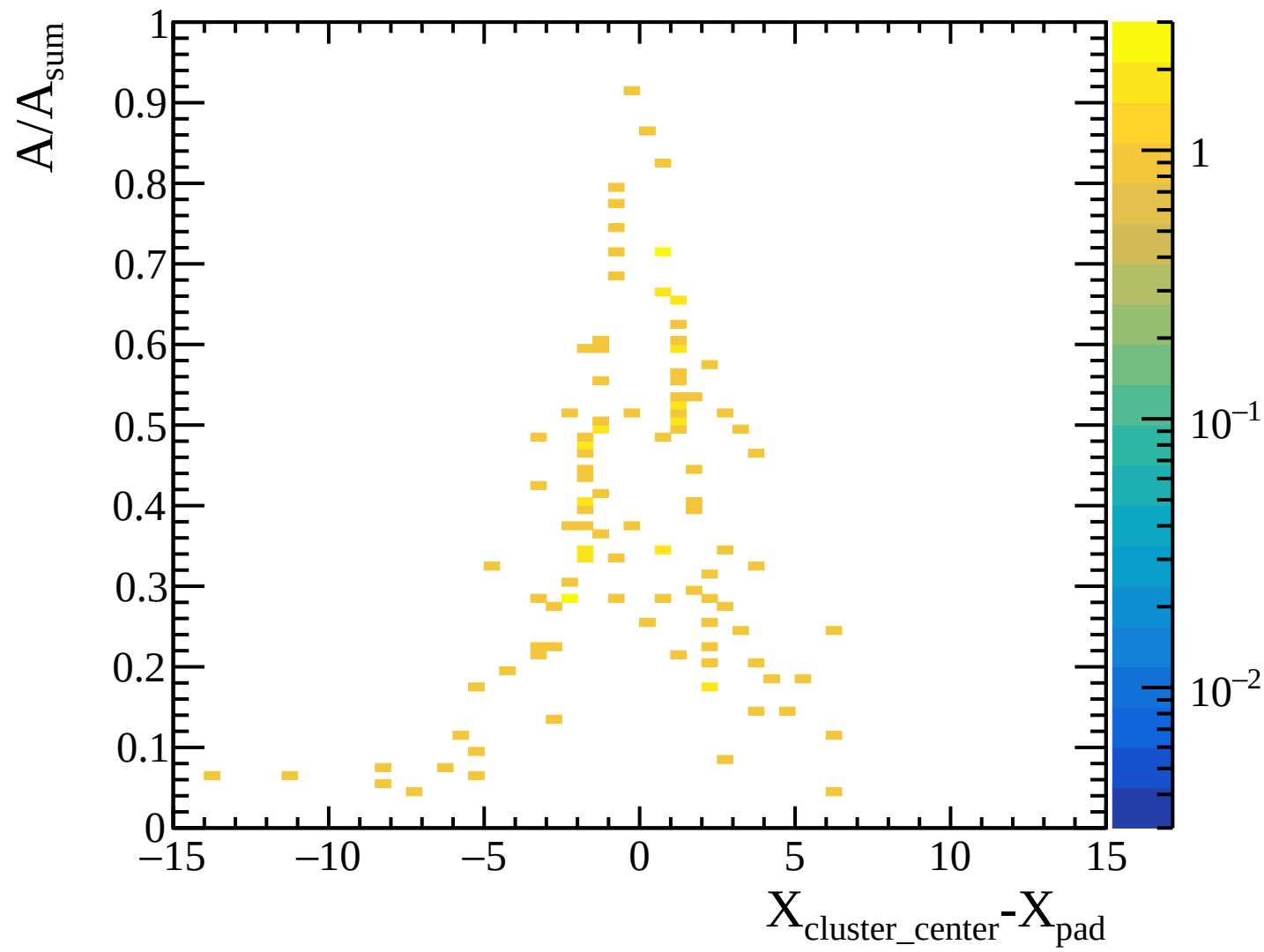
TPC transverse diffusion: layer 02 [Transverse_Diffusion_Layer02]
