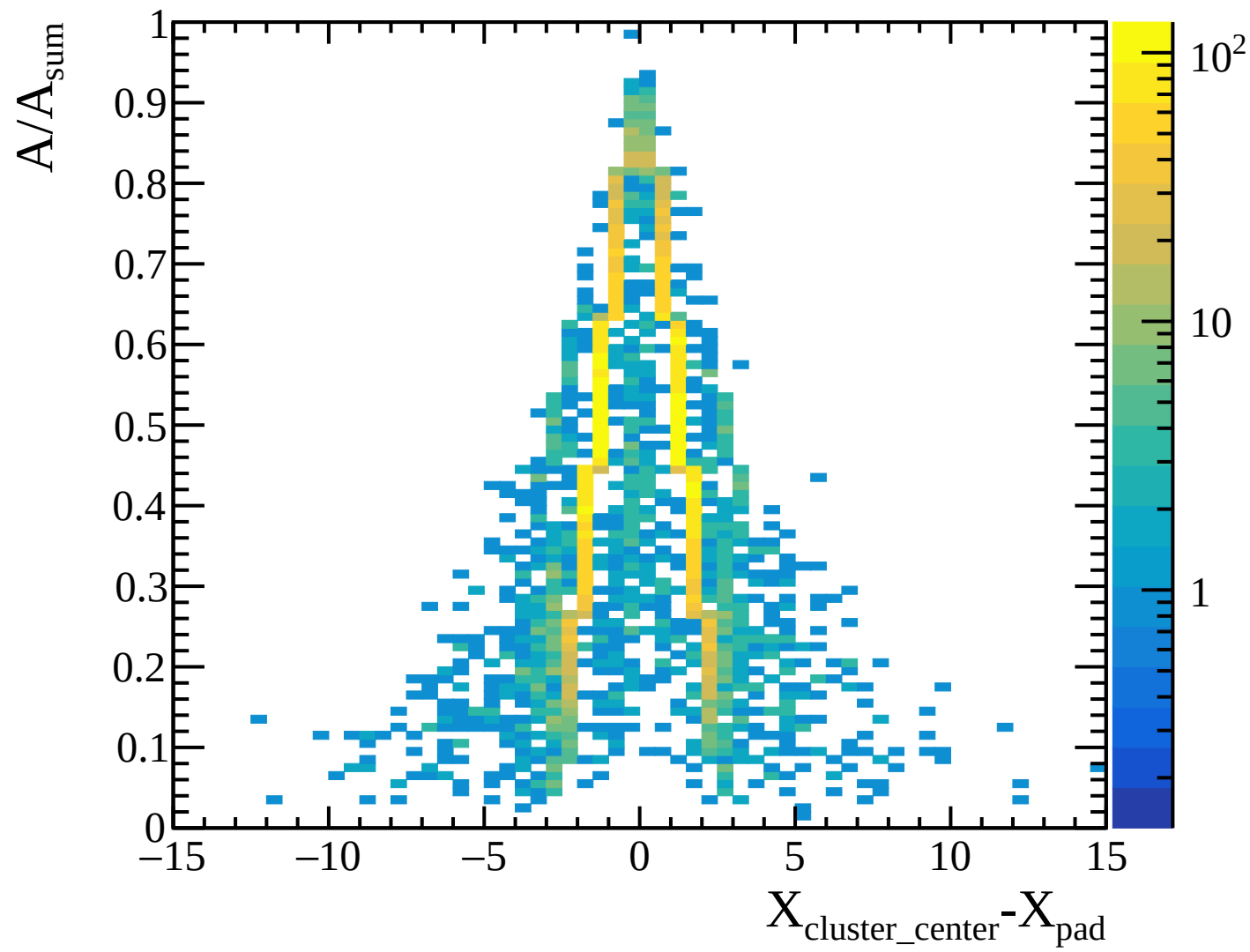
TPC transverse diffusion: layer 05 [Transverse_Diffusion_Layer05]
