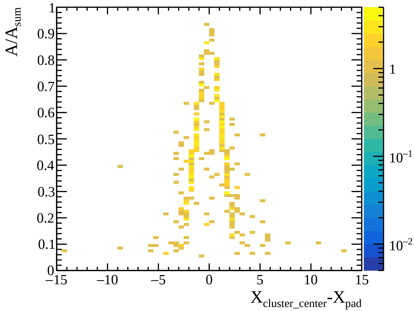
TPC transverse diffusion: layer 04 [Transverse_Diffusion_Layer04]
