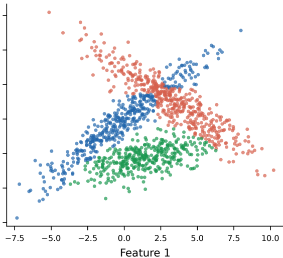
b GMM (ARI = 0.70)
