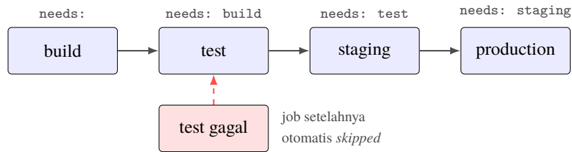
Gambar 2: Job dirangkai berurutan dengan needs: . Ketika satu job gagal, job setelahnya tidak dijalankan.
