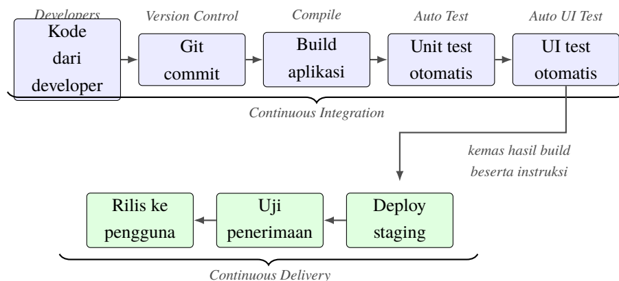
Gambar 1: Alur CI/CD: tahap continuous integration berhenti setelah pengujian otomatis, lalu continuous delivery melanjutkan sampai rilis ke pengguna.
