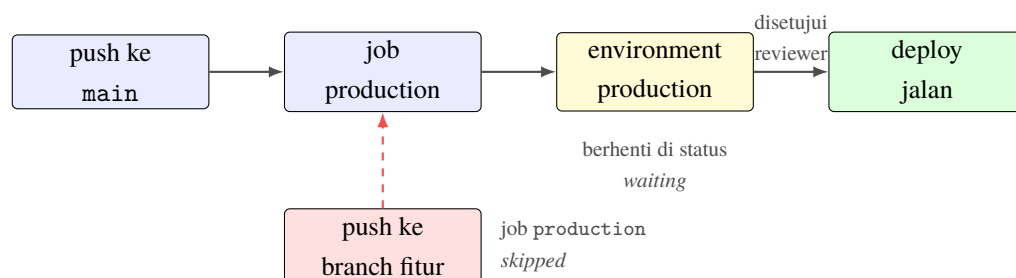
Gambar 4: Job production hanya berjalan dari main dan menunggu persetujuan reviewer pada environment. Push ke branch fitur melewatinya.
