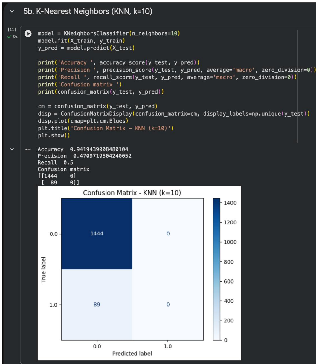
Gambar 22: Output performa KNN: Accuracy 0.9419, Precision 0.4709, Recall 0.5000, Confusion Matrix [[1444, 0], [89, 0]], identik dengan Logistic Regression dan gagal mendeteksi kelas minoritas.
