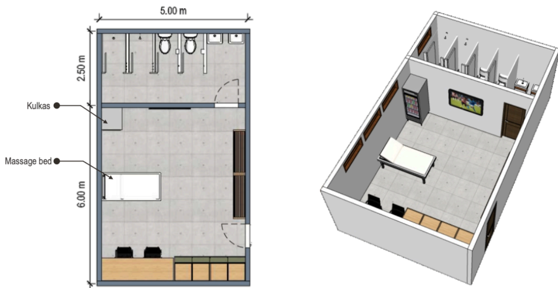
Gambar 2.10 Ilustrasi ruang ganti wasit. (Doc: Pedoman Pemenuhan Standar Venue Piala Dunia FIFA U-20)
