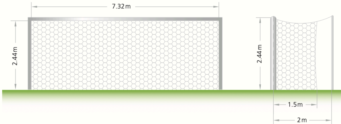
Gambar 2.3 Ukuran gawang permainan.
