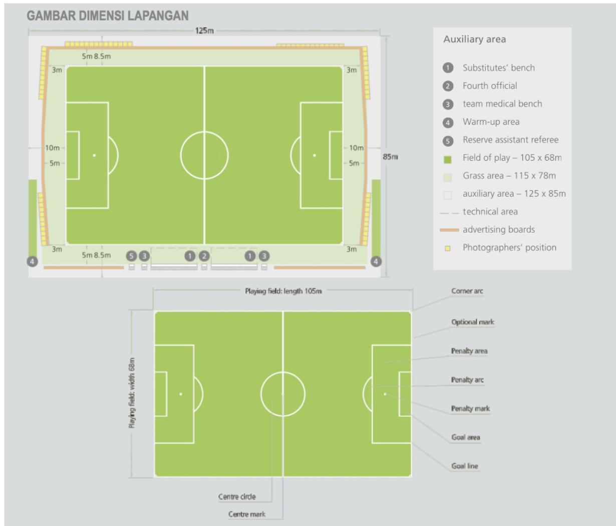
Gambar 2.2 Detail dimensi lapangan.
