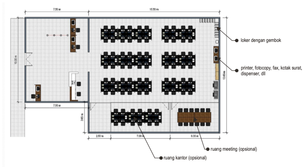
Gambar 3.1 Ilustrasi media center .
