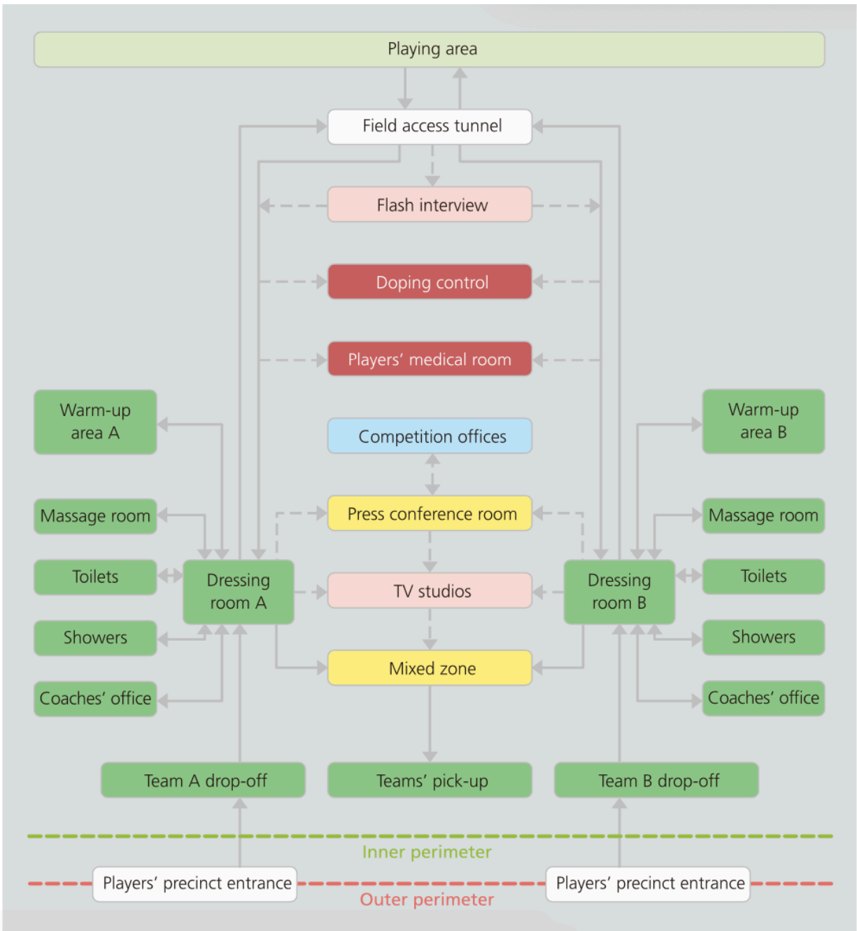
Gambar 2.13 Referensi alur pemain.
