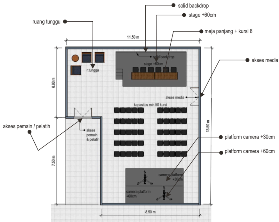
Gambar 3.2 Ilustrasi ruang konferensi pers. (Doc: Pedoman Pemenuhan Standar Venue Piala Dunia FIFA U-20)
