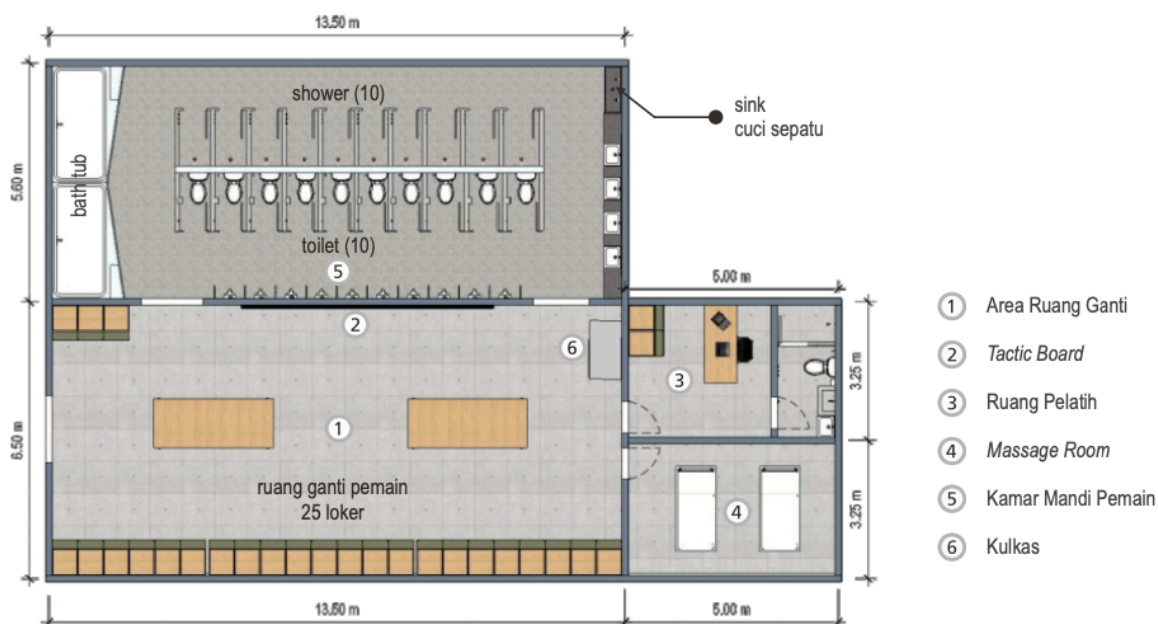
Gambar 2.9 Ilustrasi ruang ganti tim & pelatih. (Doc: Pedoman Pemenuhan Standar Venue Piala Dunia FIFA U-20)
