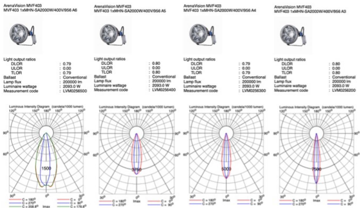
Gambar 2.7 Spesifikasi lampu stadion GBLA.
