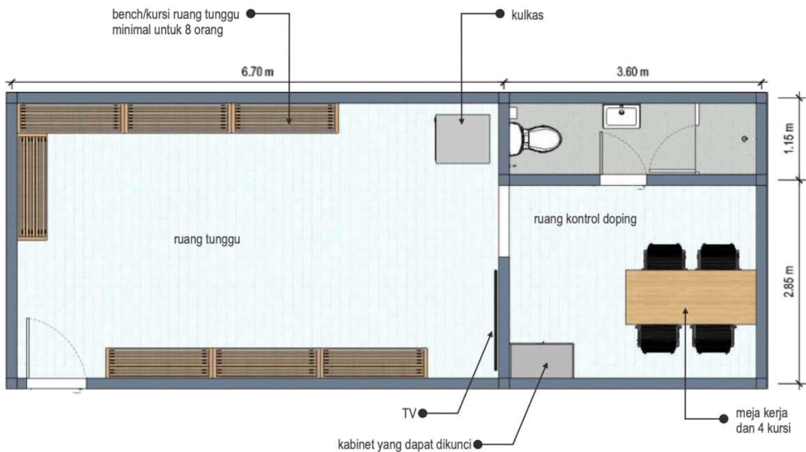
Gambar 2.12 Ilustrasi ruang doping. (Doc: Pedoman Pemenuhan Standar Venue Piala Dunia FIFA U-20)
