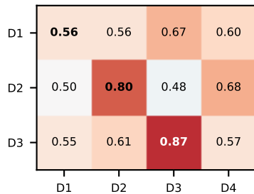
PCA
