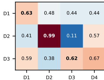
kNN
