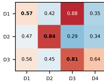
CLAD
