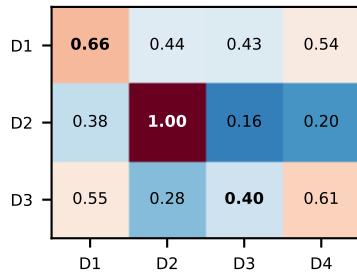
Mahalanobis
