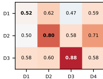
AE
