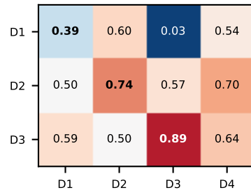
OCSVM
