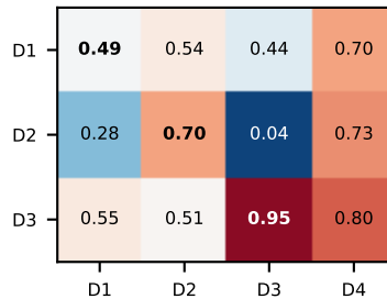
IF
