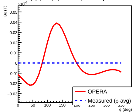
B_\phi (T) vs \phi ( r=30 cm, z=0 cm)
