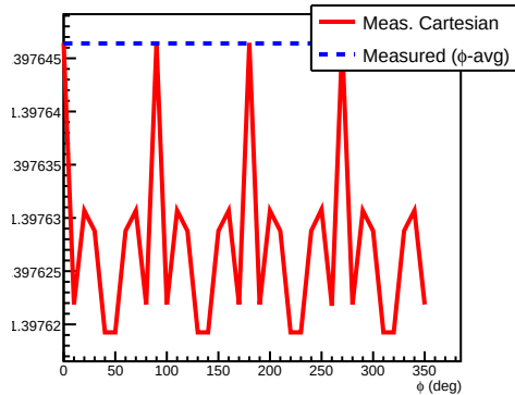
B_z (T) vs \phi ( r=30 cm, z=0 cm)
