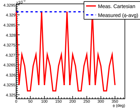
B_r (T) vs \phi ( r=30 cm, z=0 cm)
