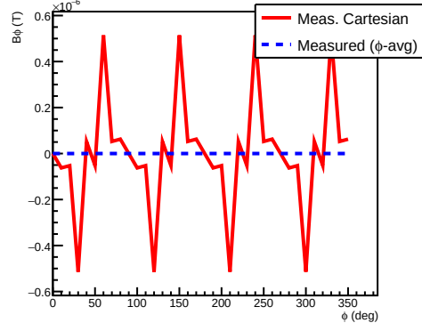
B_\phi (T) vs \phi ( r=30 cm, z=0 cm)
