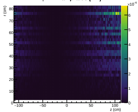
B_\phi m=1 amplitude [mT]
