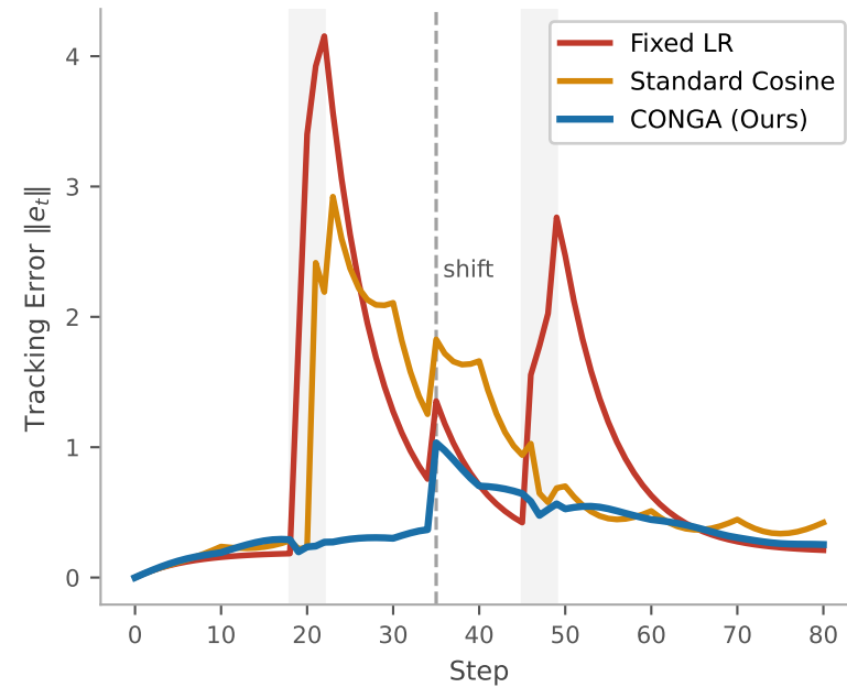
(d) Tracking Error Comparison
