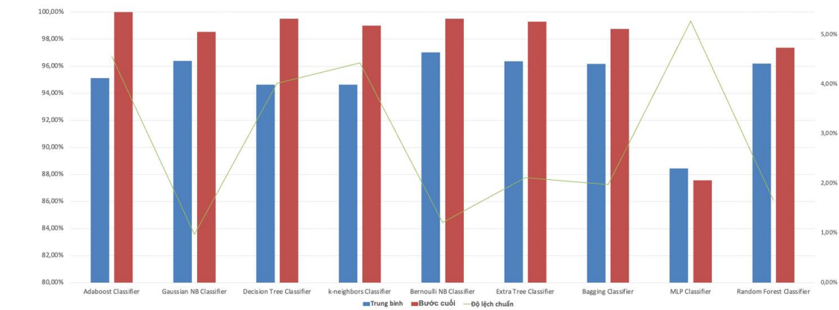
Hình 3. Biểu đồ thể hiện tương quan kết quả giữa 9 giải thuật
