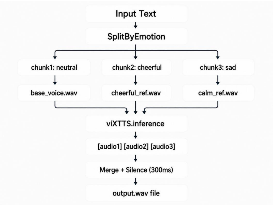
Fig. 1. Workflow of the Proposed Emotion-Based Speech Synthesis System | Fig. 1. Werkvloei van die voorgestelde emosie-gebaseerde spraaksintese stelsel
