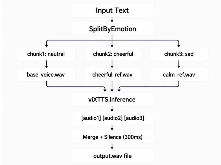
Fig. 1. Workflow of the Proposed Emotion-Based Speech Synthesis System | Hình 1. Quy trình làm việc của Hệ thống tổng hợp giọng nói dựa trên cảm xúc được đề xuất
