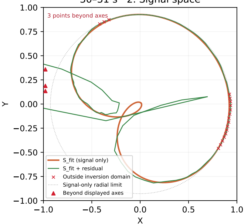
30-31 s · 2. Signal space
