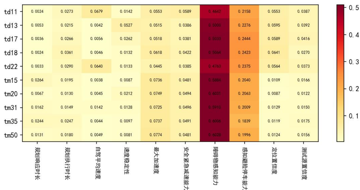
图 11 各指标对无人车障碍度热图
