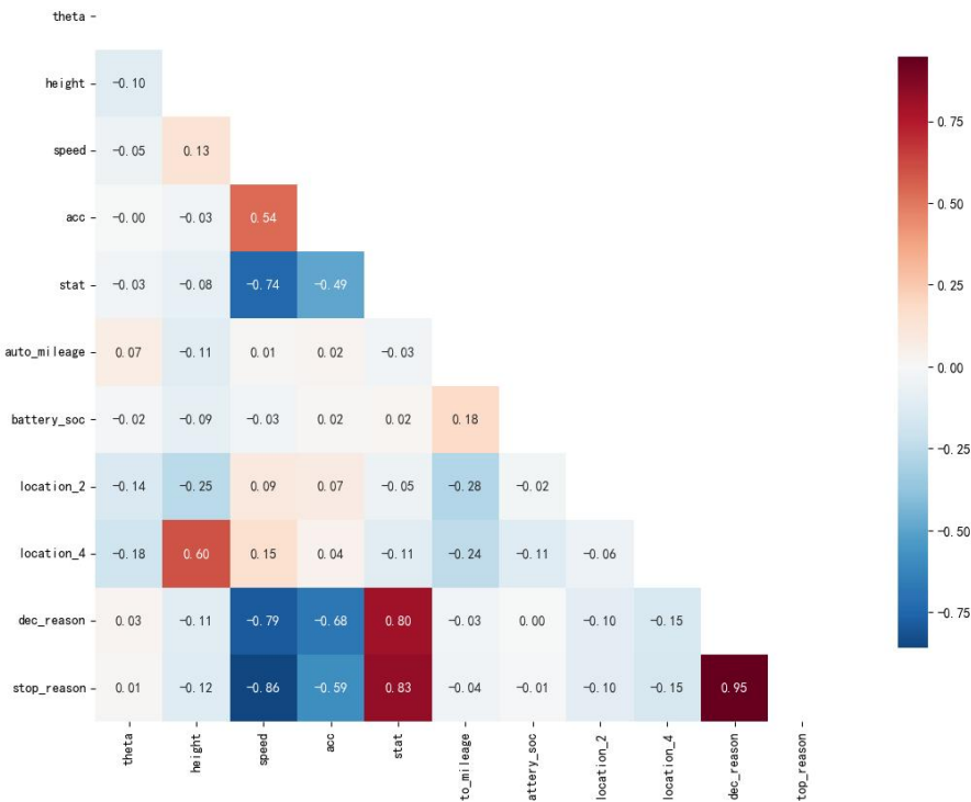
图 6 连续型变量相关性热图
