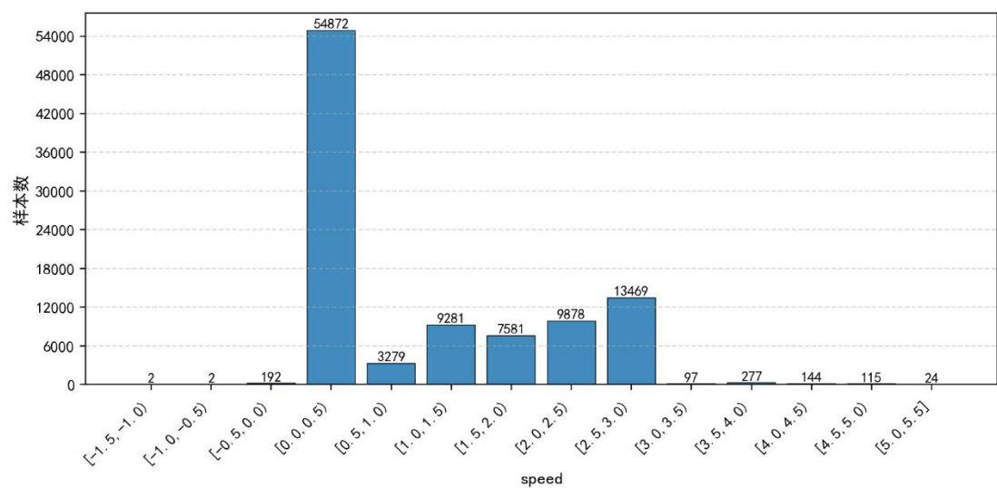
图 5 速度取值统计直方图
