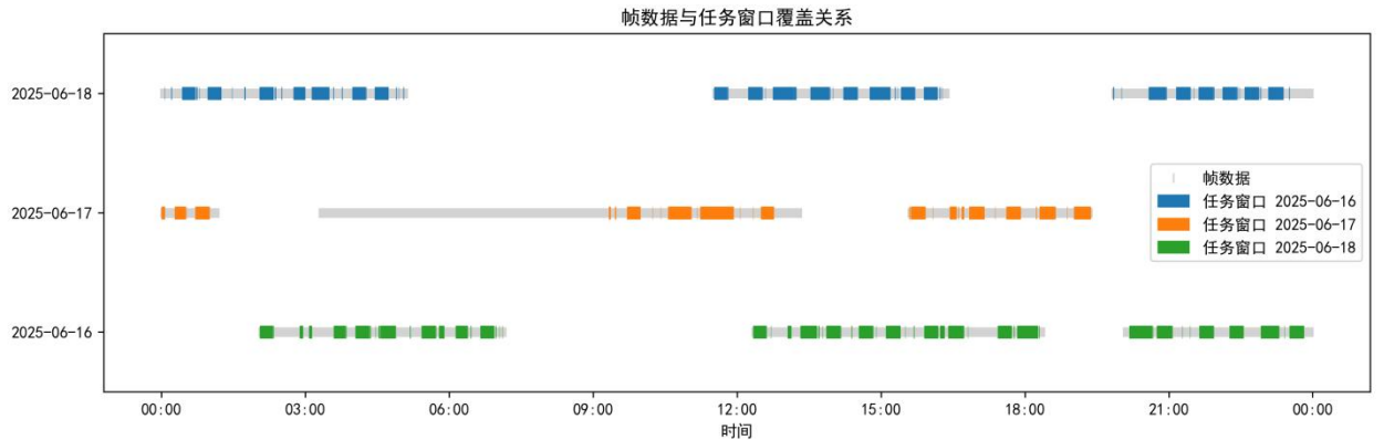
图 2 样本时间窗口可视化
