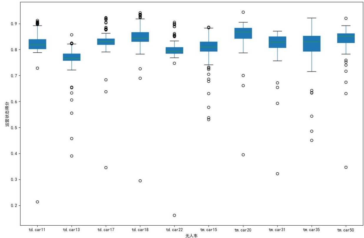
图 8 各无人车运营得分箱线图
