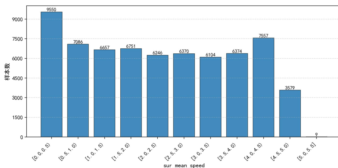
图 13 周围车辆平均速度取值统计直方图
