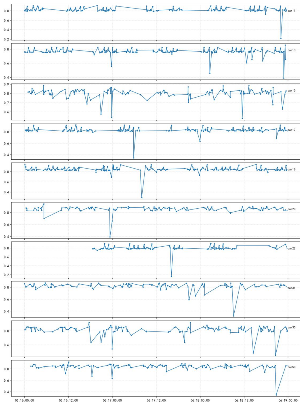
图 9 无人车运营得分对比折线图
