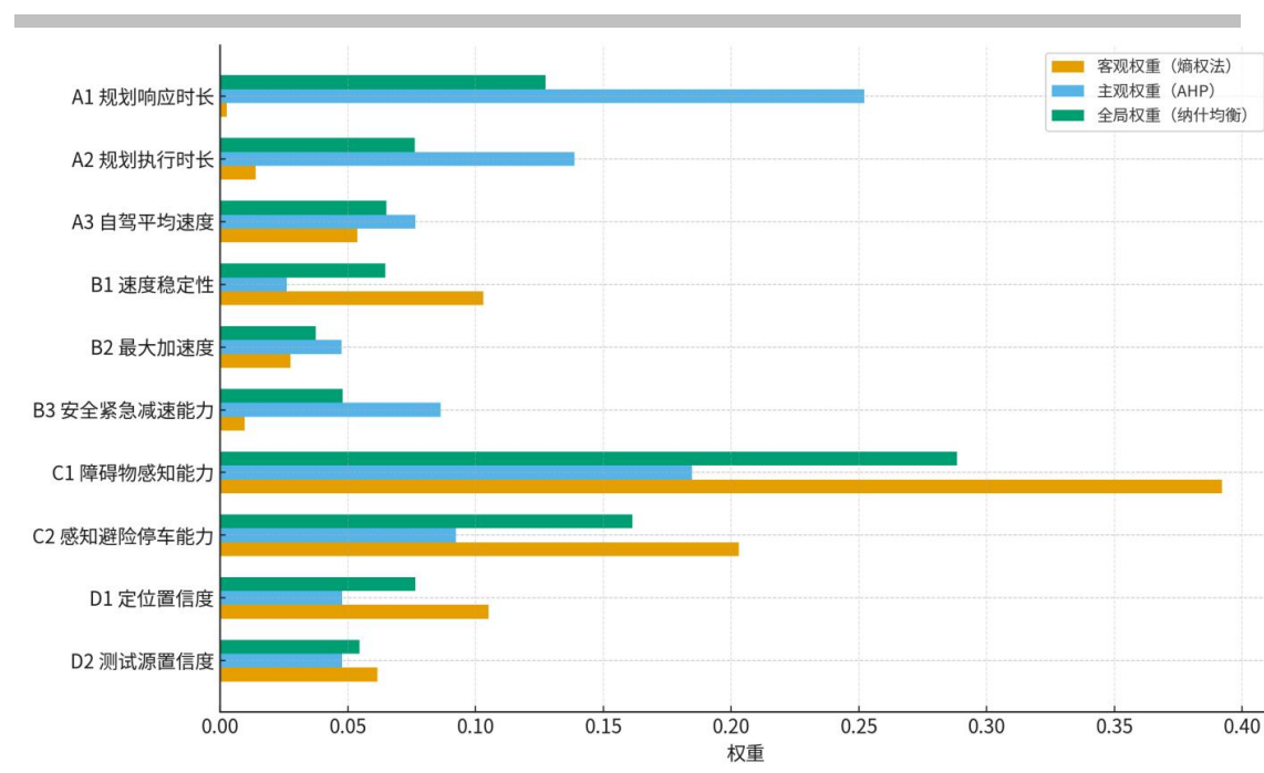
图 7 权重对比横向条形图
