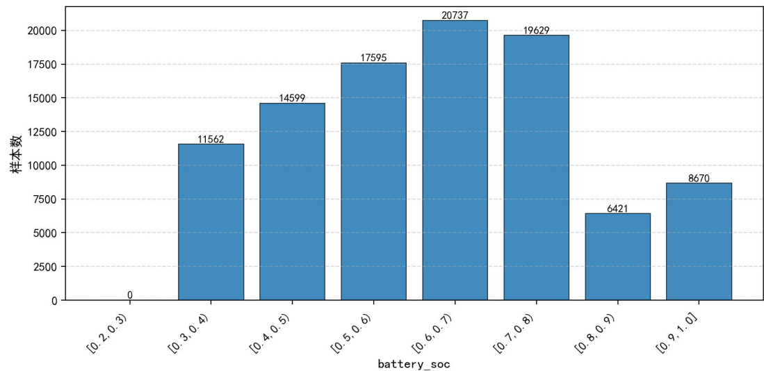
图 3 电量取值统计直方图
