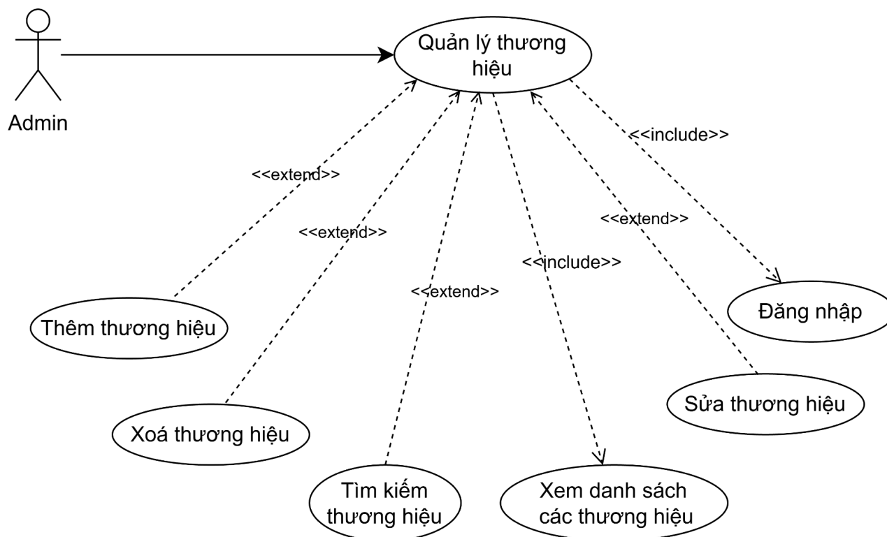
Hình 2.15. Biểu đồ phân rã Use Case UC14 - Quản lý thương hiệu
