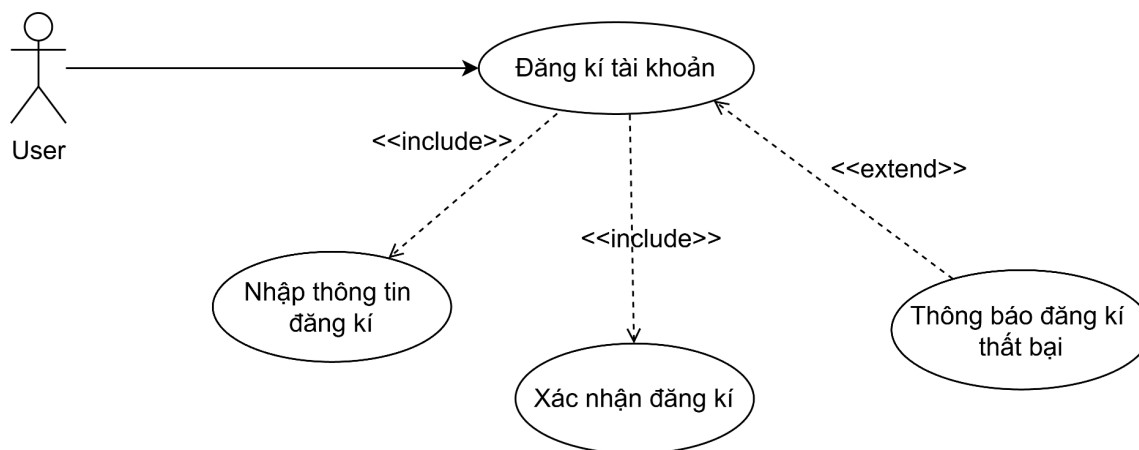
Hình 2.2. Biểu đồ phân rã Use Case UC01 - Đăng ký tài khoản
