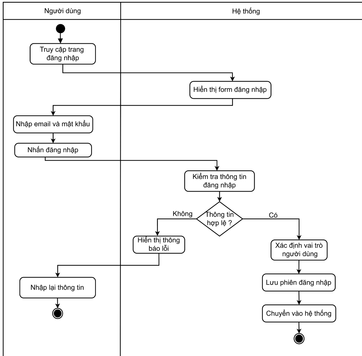
Hình 2.32. Biểu đồ hoạt động đăng nhập tài khoản
