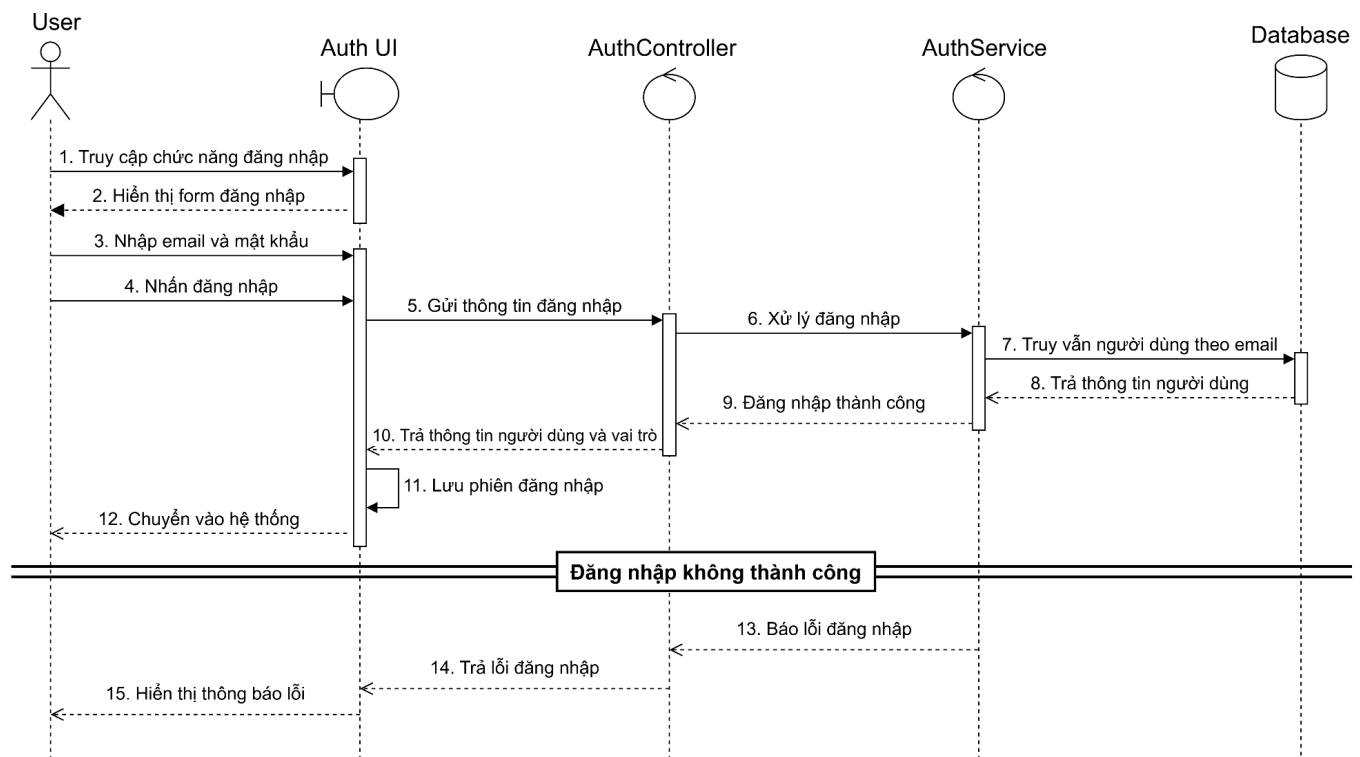
Hình 2.22. Biểu đồ trình tự Đăng nhập tài khoản
