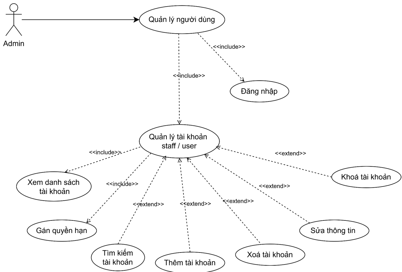
Hình 2.12. Biểu đồ phân rã Use Case UC11 - Quản lý người dùng
