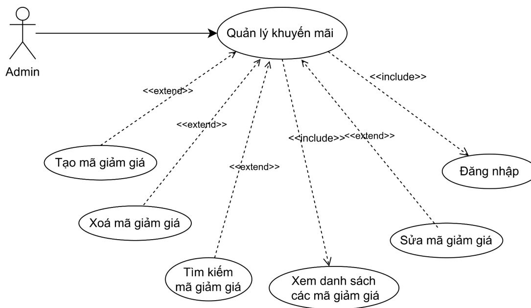
Hình 2.17. Biểu đồ phân rã Use Case UC16 - Quản lý khuyến mãi
