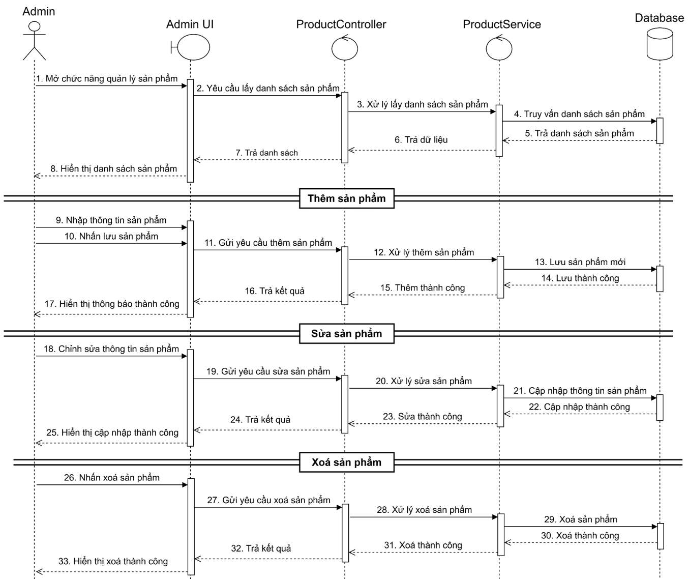
Hình 2.27. Biểu đồ trình tự Quản lý sản phẩm
