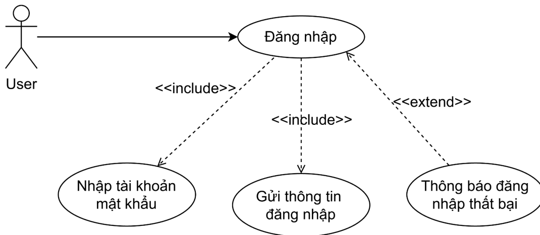
Hình 2.3. Biểu đồ phân rã Use Case UC02 - Đăng nhập tài khoản
