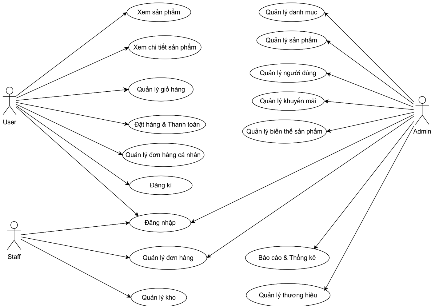
Hình 2.19. Biểu đồ Use Case tổng quát
