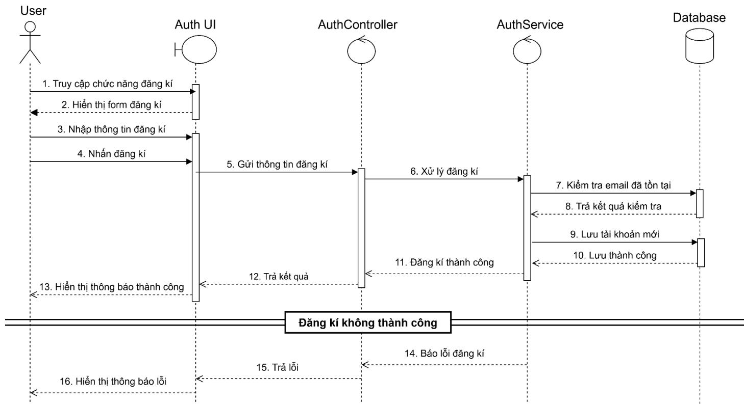
Hình 2.21. Biểu đồ trình tự Đăng kí tài khoản
