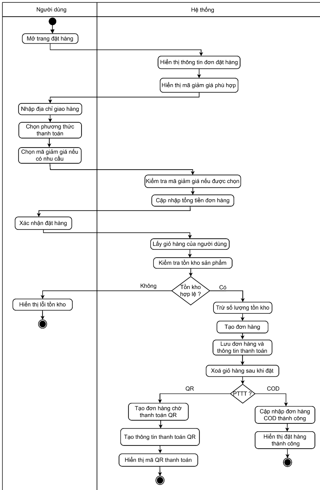
Hình 2.34. Biểu đồ hoạt động Đặt hàng và thanh toán
