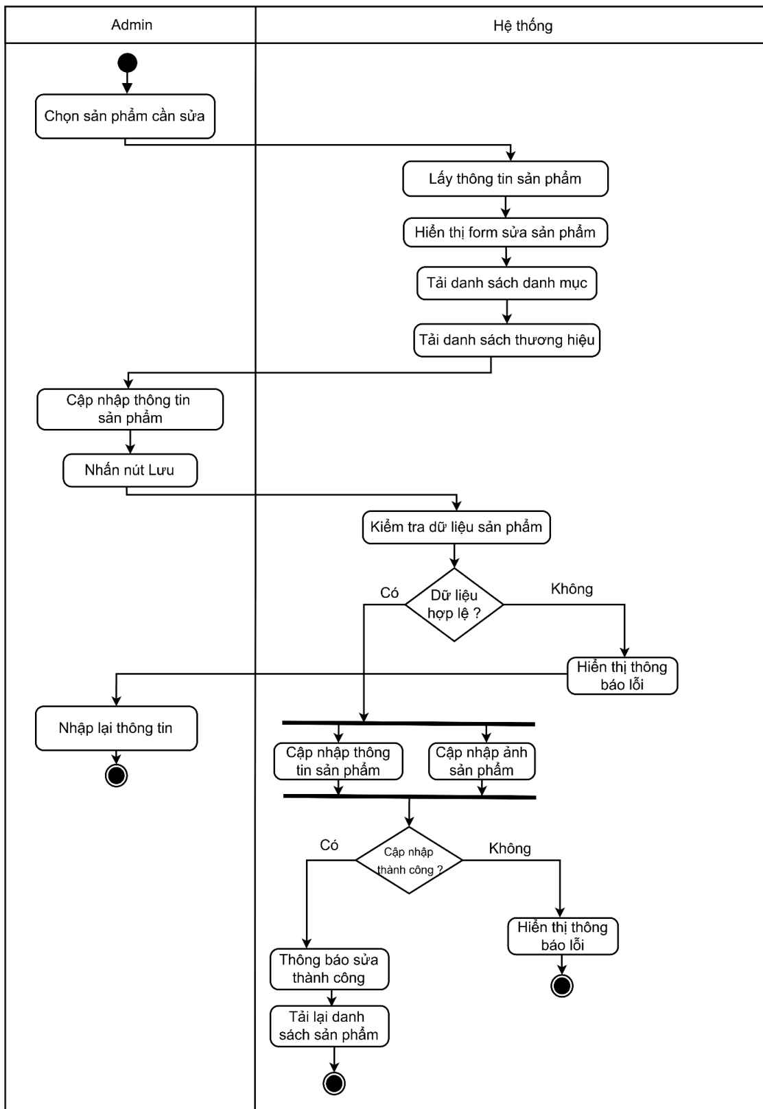
Hình 2.36. Biểu đồ hoạt động Sửa sản phẩm
