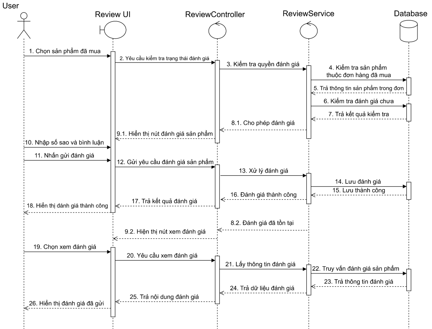
Hình 2.26. Biểu đồ trình tự Đánh giá sản phẩm
