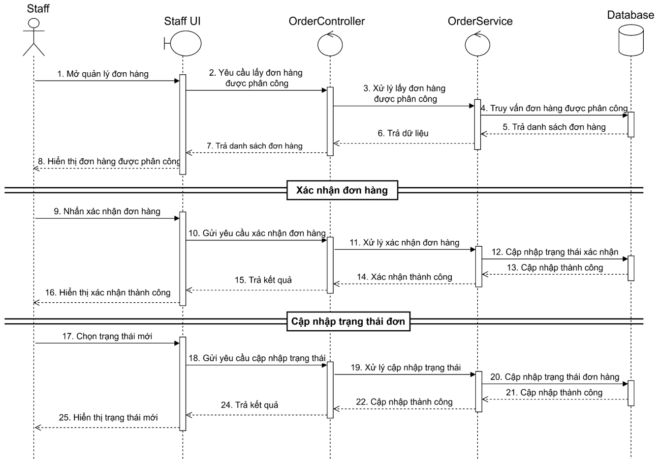
Hình 2.30. Biểu đồ trình tự Quản lý đơn hàng
