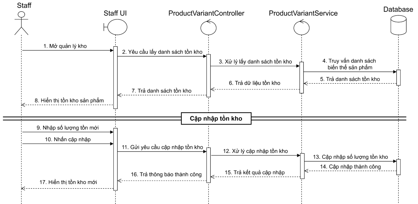
Hình 2.29. Biểu đồ trình tự Quản lý kho
