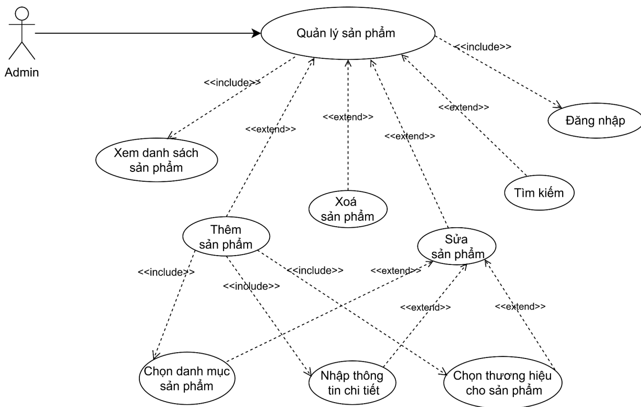
Hình 2.13. Biểu đồ phân rã Use Case UC12 - Quản lý sản phẩm
