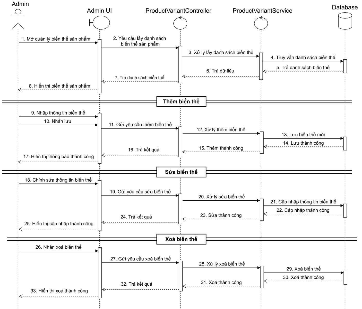
Hình 2.28. Biểu đồ trình tự Quản lý biến thể sản phẩm
