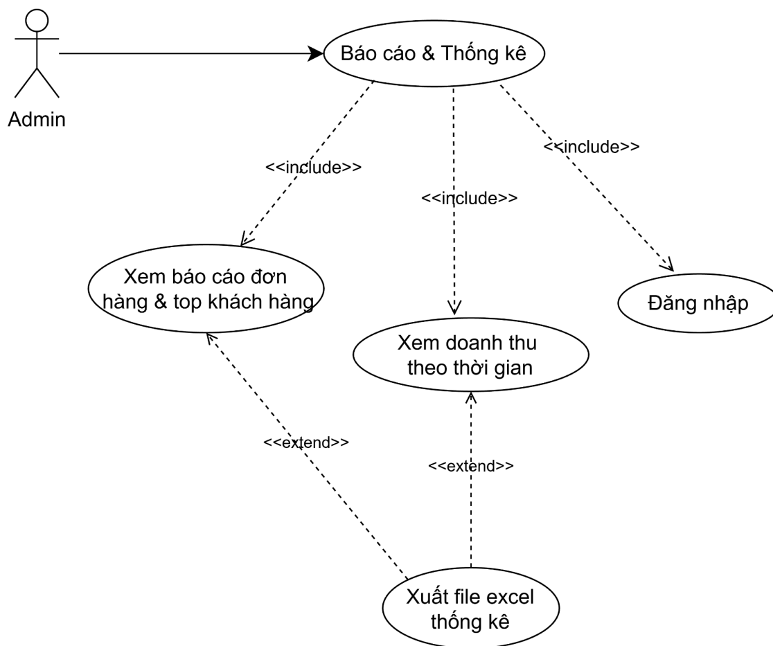
Hình 2.18. Biểu đồ phân rã Use Case UC17 - Báo cáo và thống kê
