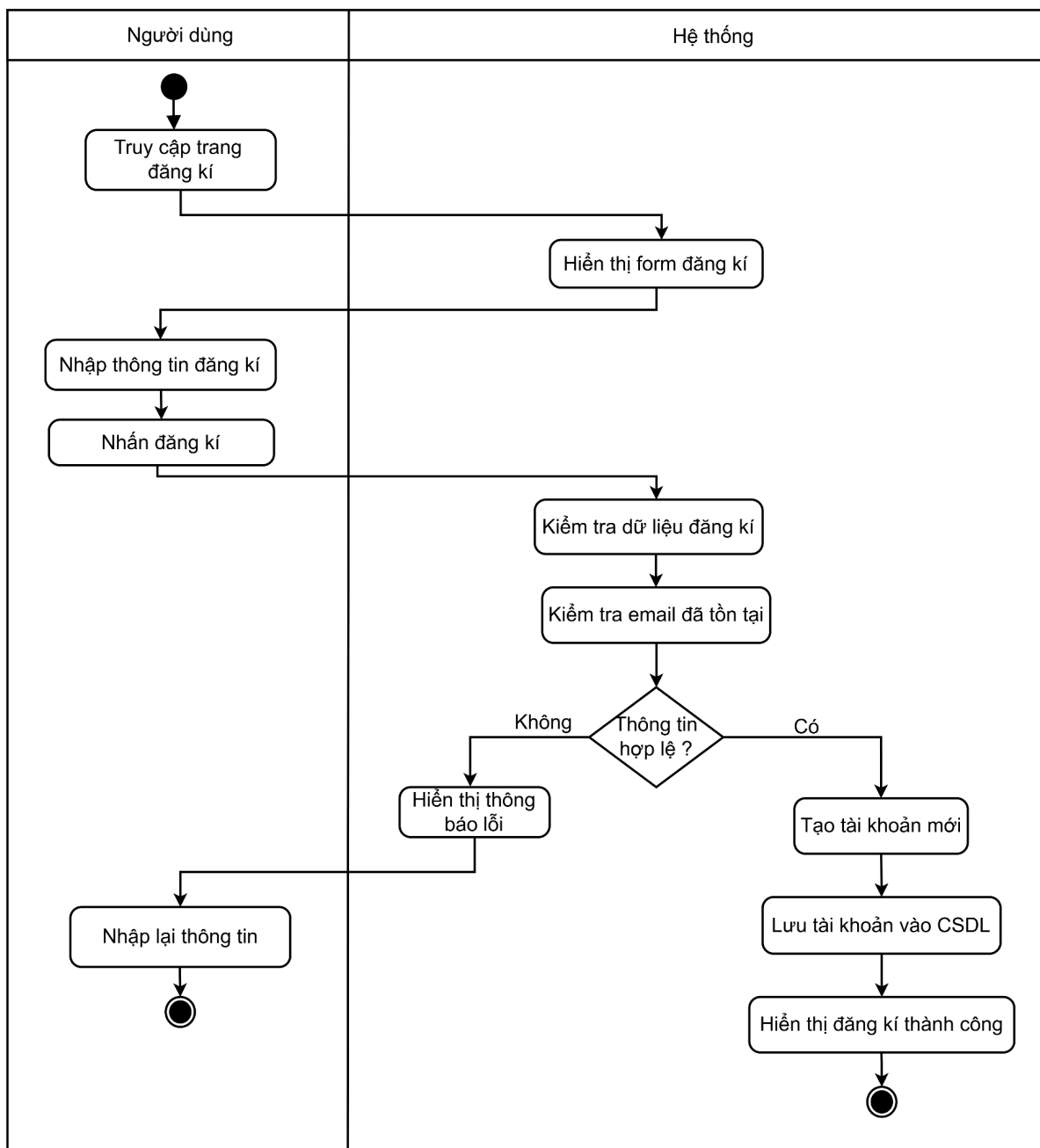
Hình 2.31. Biểu đồ hoạt động đăng kí tài khoản
