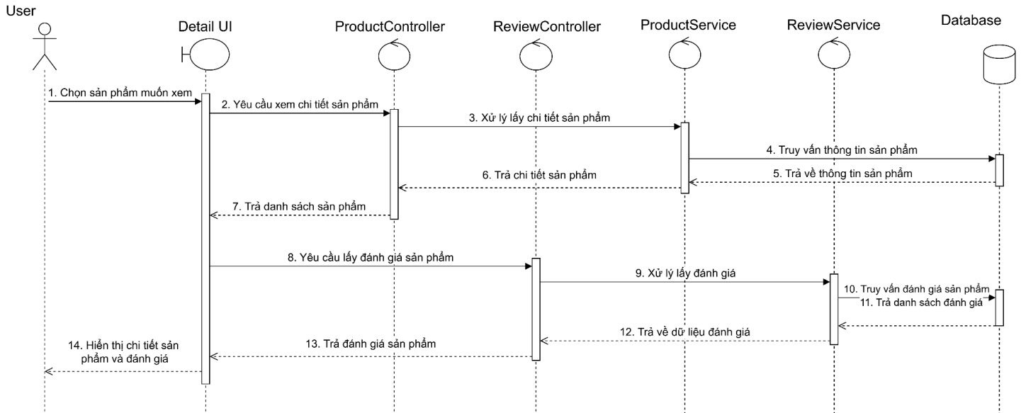
Hình 2.23. Biểu đồ trình tự Xem chi tiết sản phẩm
