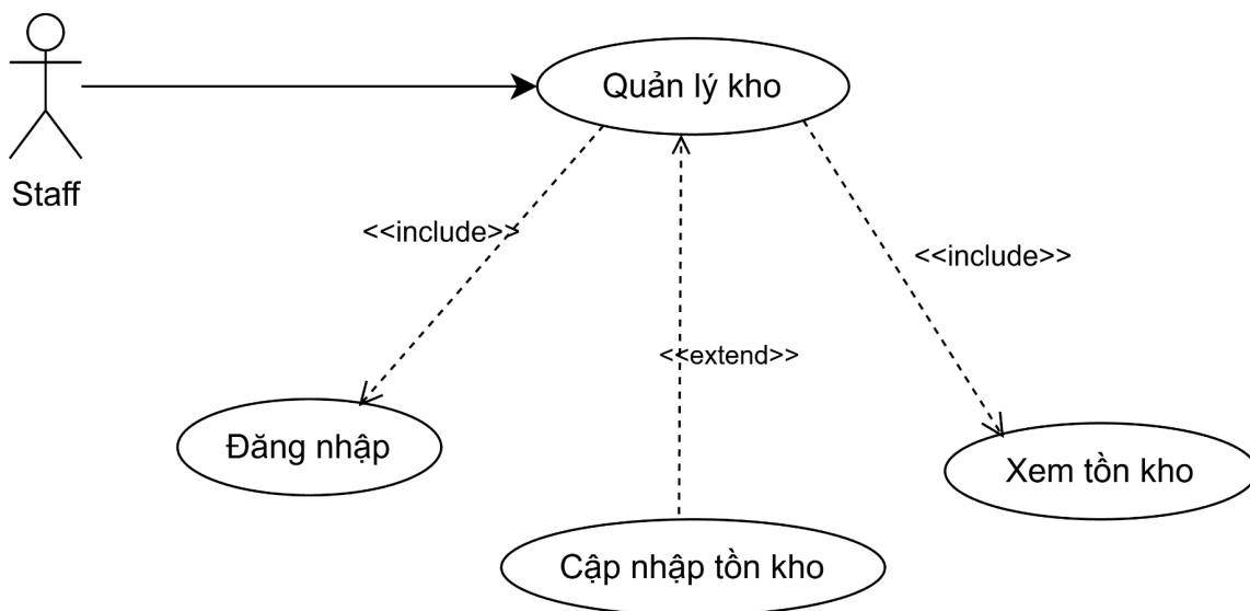
Hình 2.11. Biểu đồ phân rã Use Case UC10 - Quản lý kho
