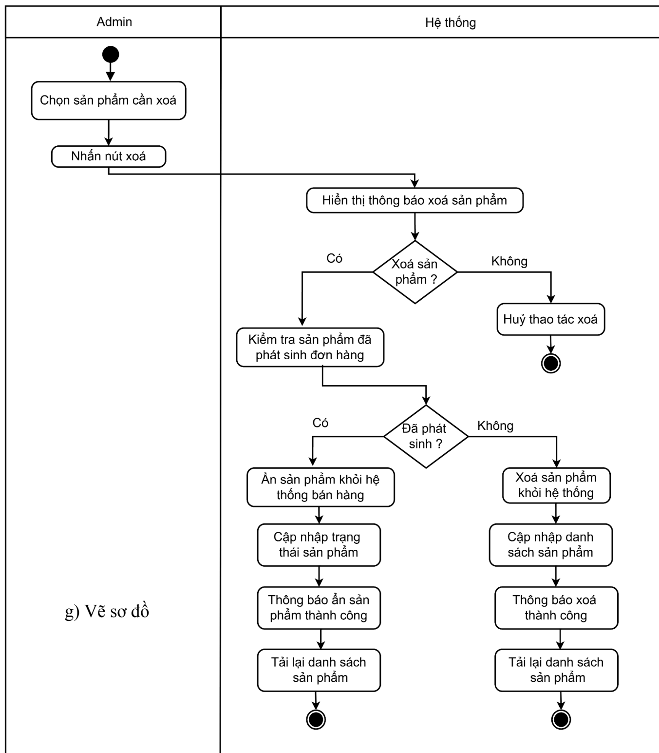
Hình 2.37. Biểu đồ hoạt động Xoá sản phẩm
