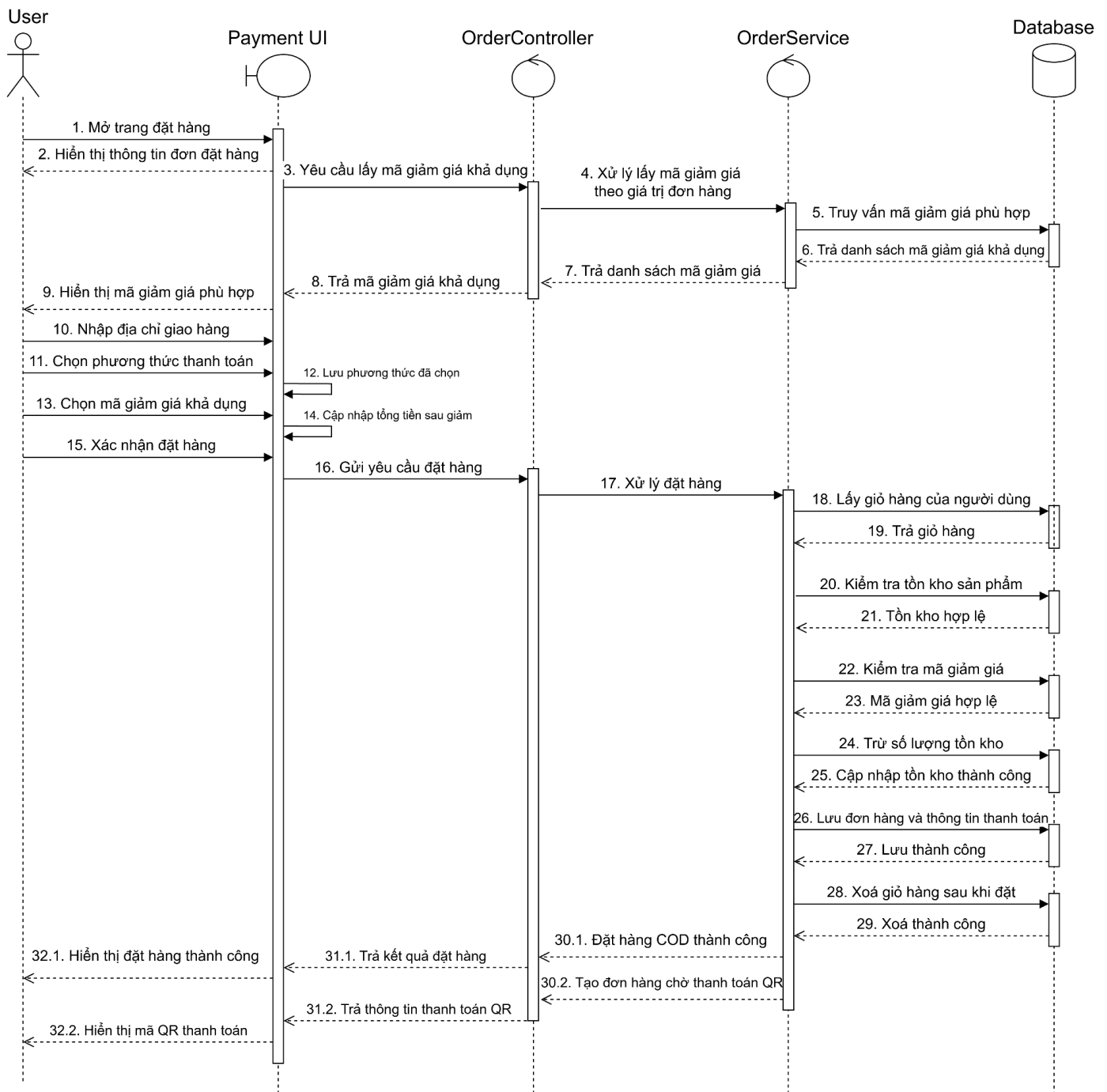
Hình 2.25. Biểu đồ trình tự Đặt hàng và thanh toán
