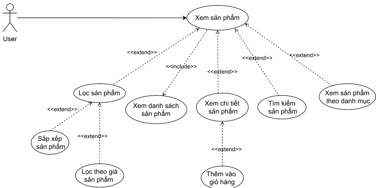
Hình 2.4. Biểu đồ phân rã Use Case UC03 - Xem sản phẩm
