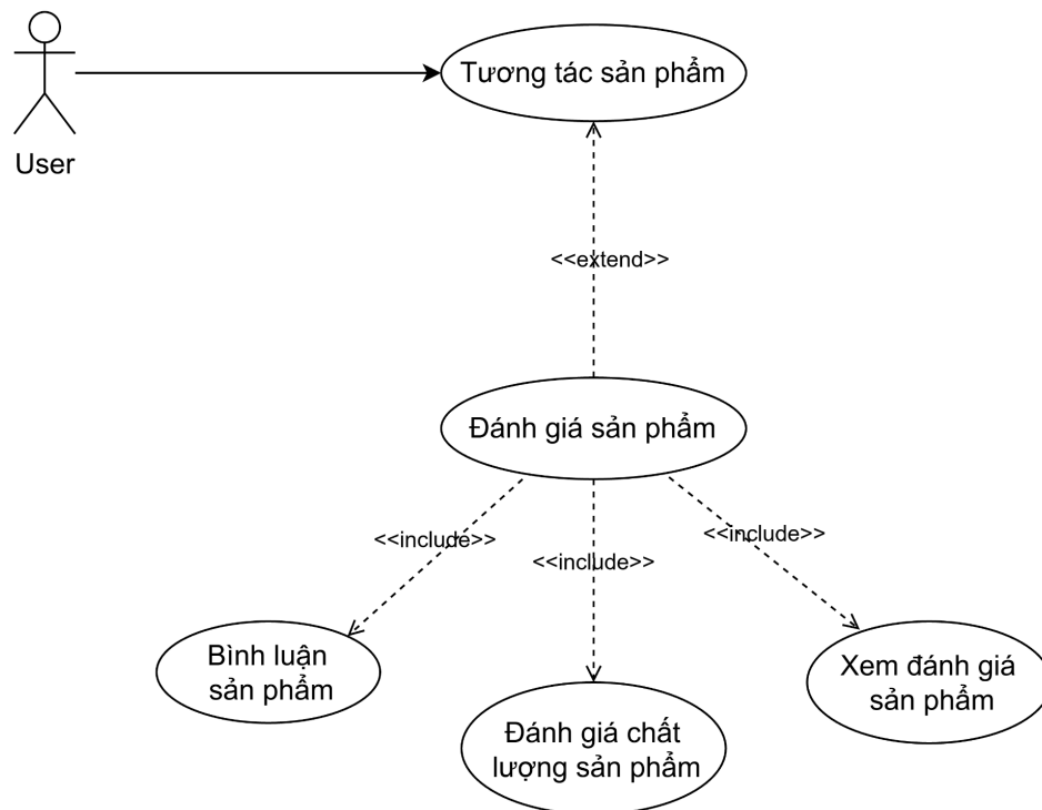
Hình 2.9. Biểu đồ phân rã Use Case UC08 - Đánh giá và tương tác sản phẩm
