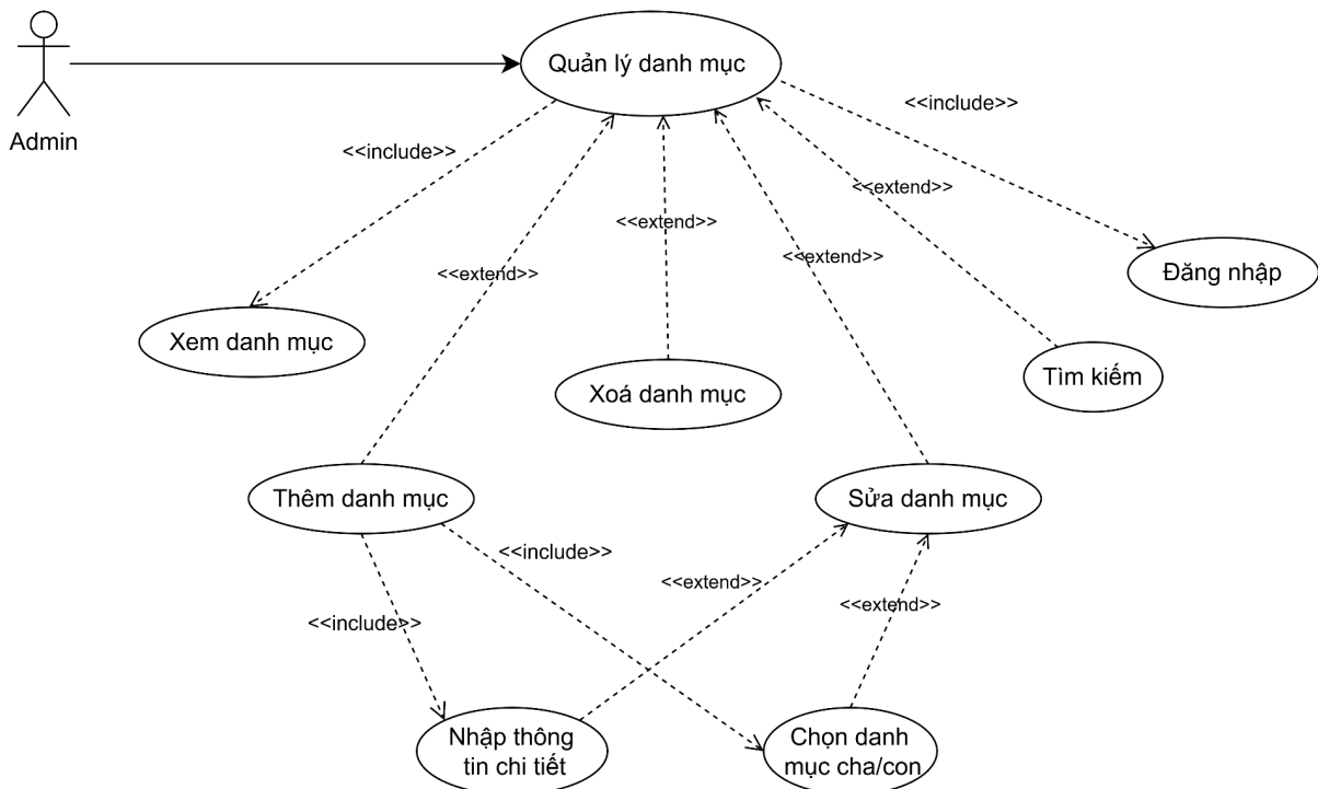
Hình 2.14. Biểu đồ phân rã Use Case UC13 - Quản lý danh mục
