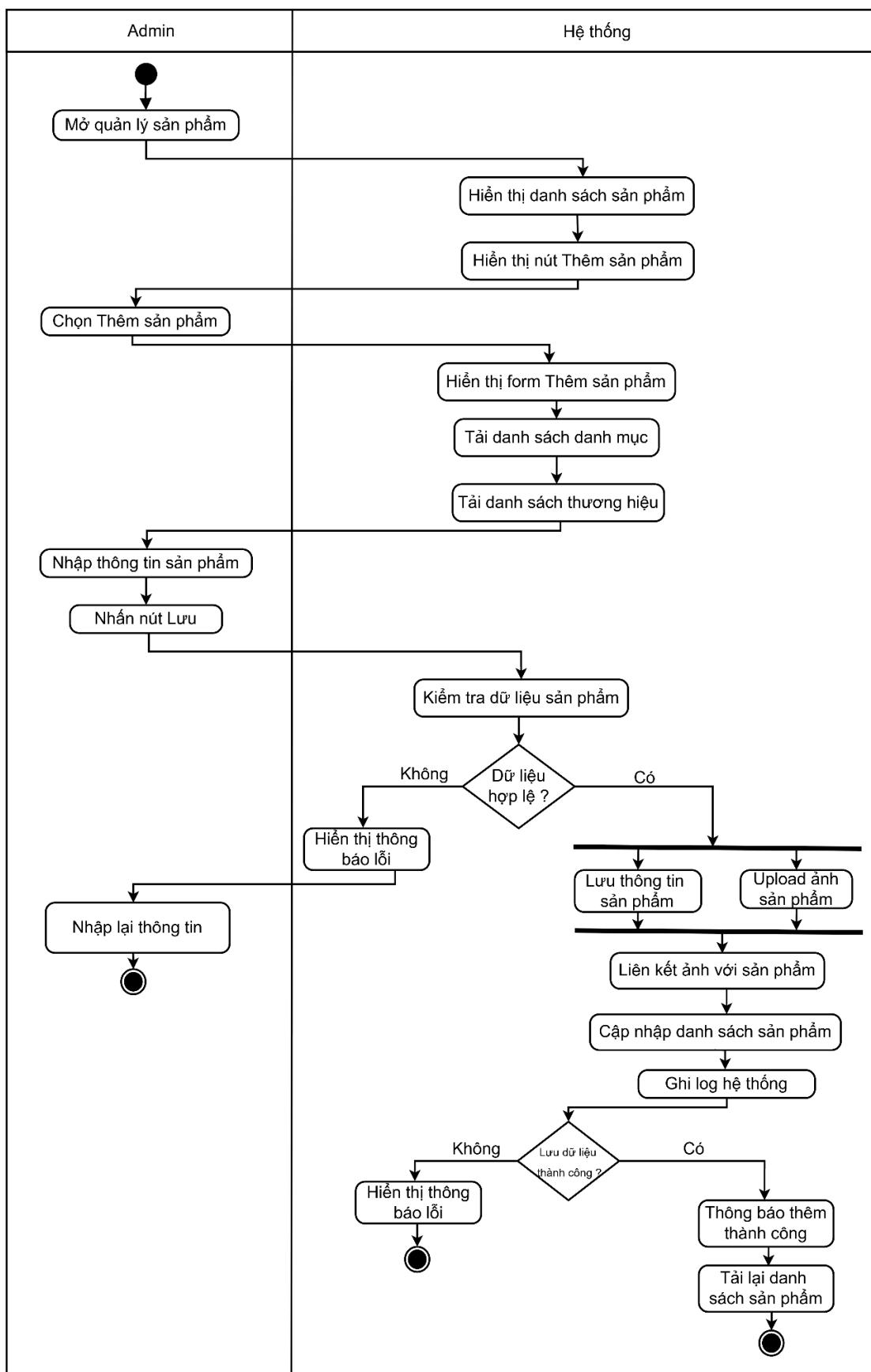
Hình 2.35. Biểu đồ hoạt động Thêm sản phẩm
