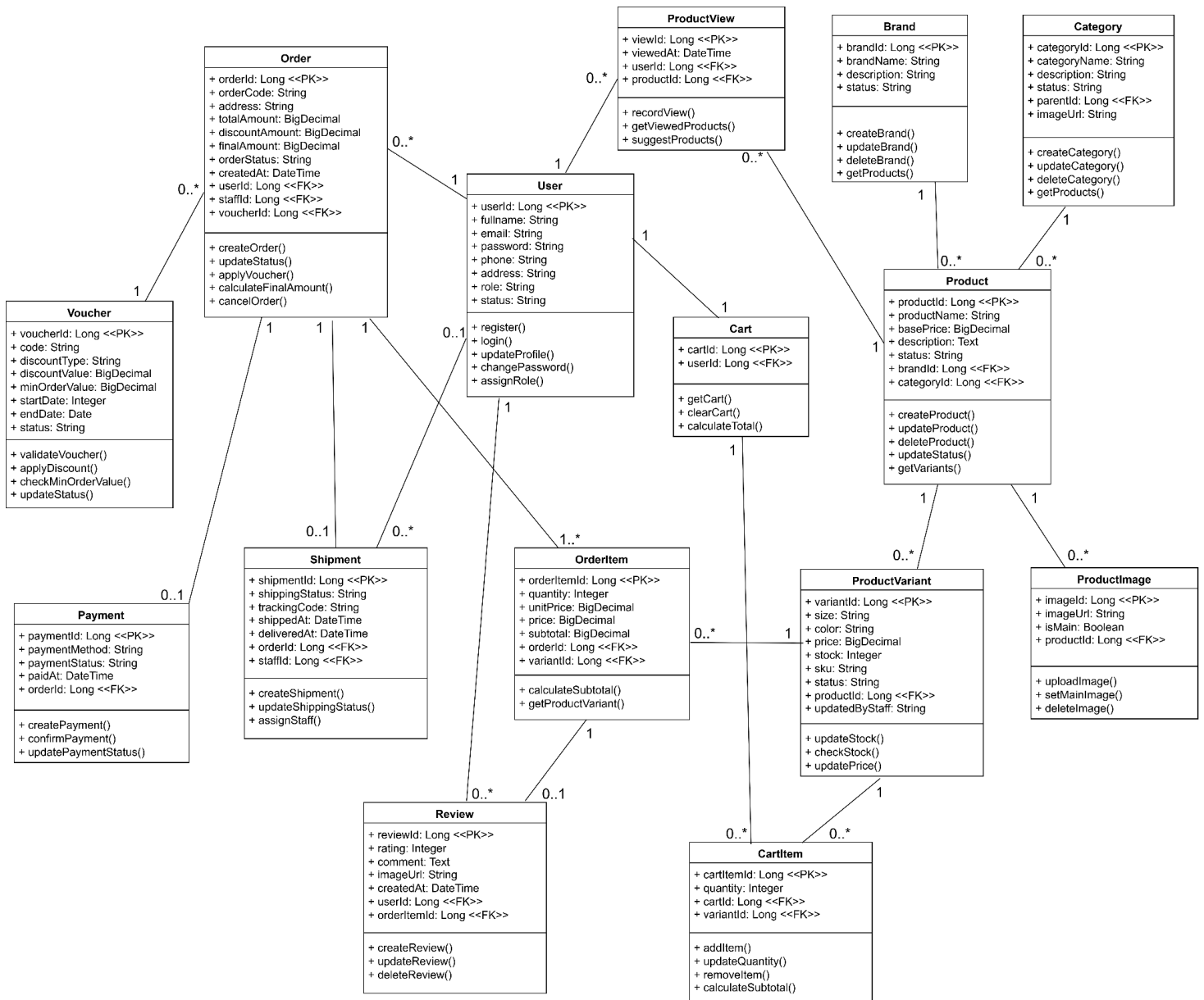
Hình 2.20. Mô hình lớp của hệ thống
