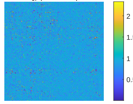
(j) |Residual|
