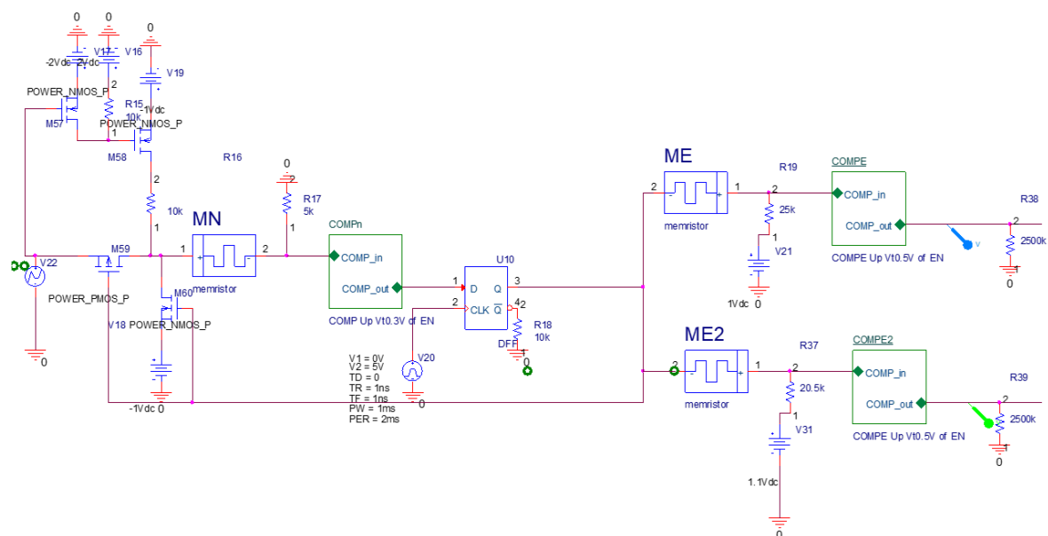
图 2-8 EN单元电路原理图
