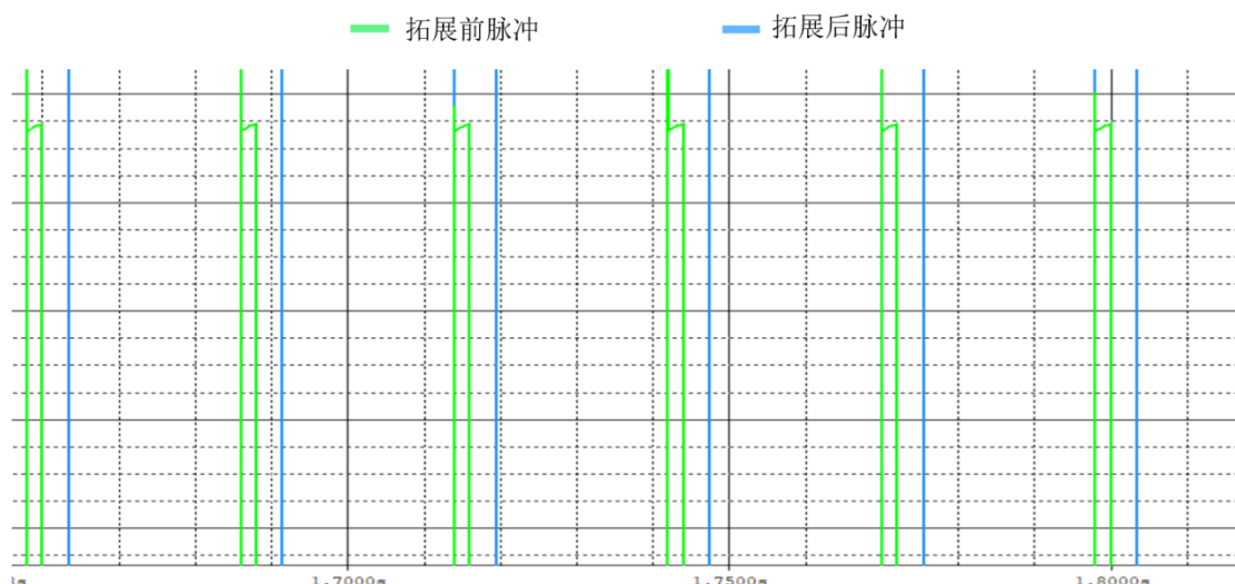
图 2-9 EN单元脉宽拓展电路特性
