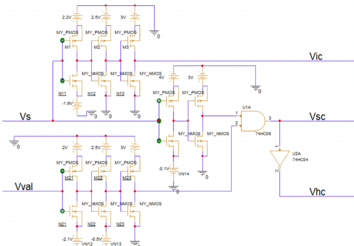
图 2-3 SJ单元电路原理图
