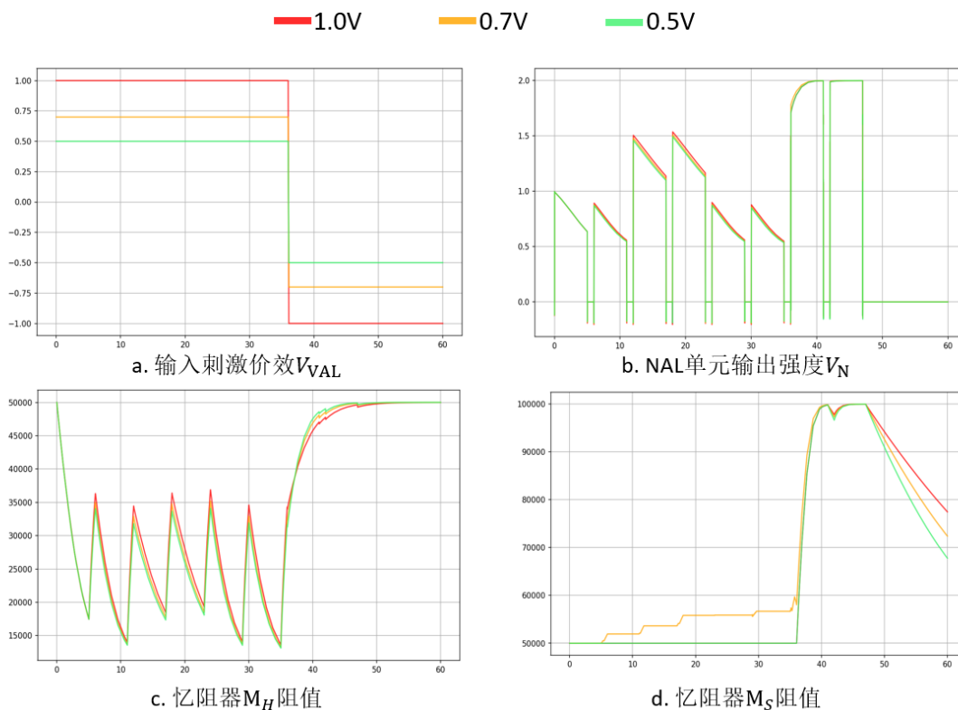
图 2-7 不同刺激价效下的电路特性
