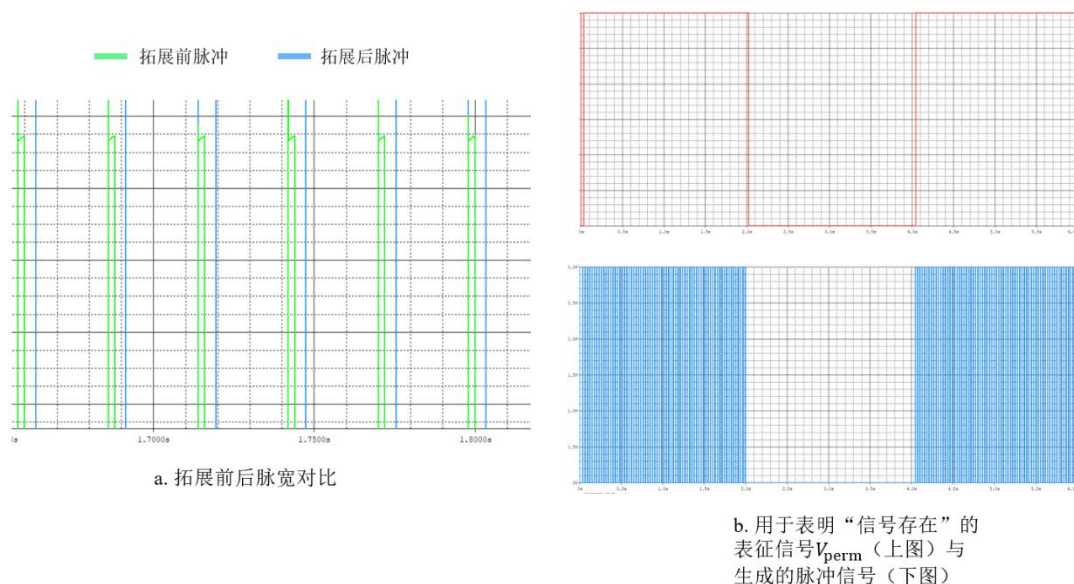
图 2-8 EN单元电路特性
