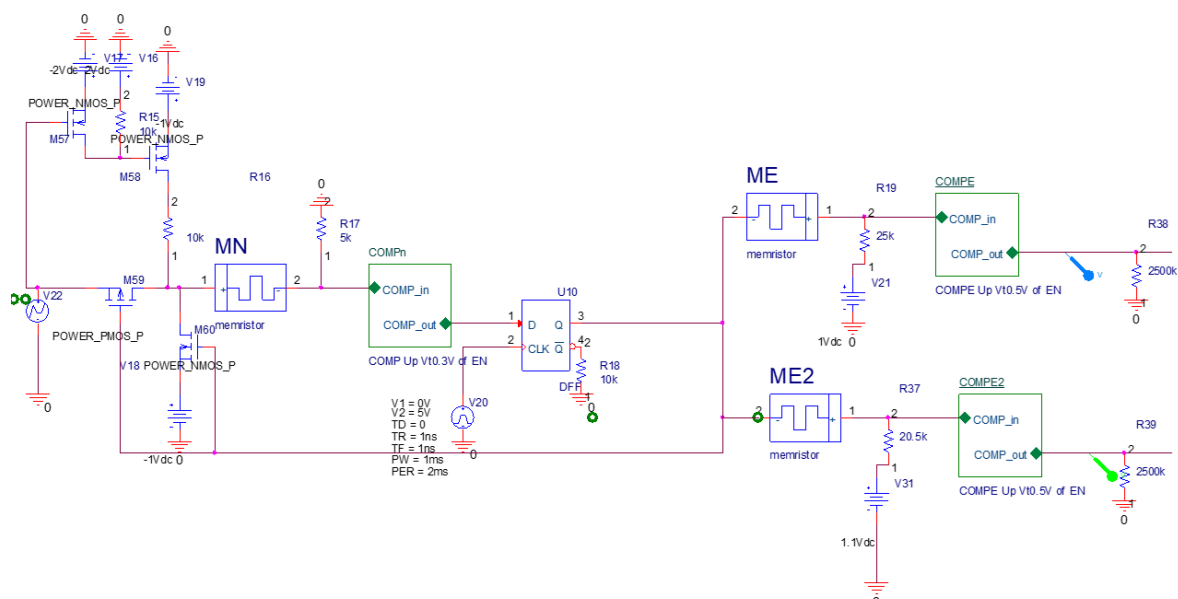
图 2-9 EN单元电路图
