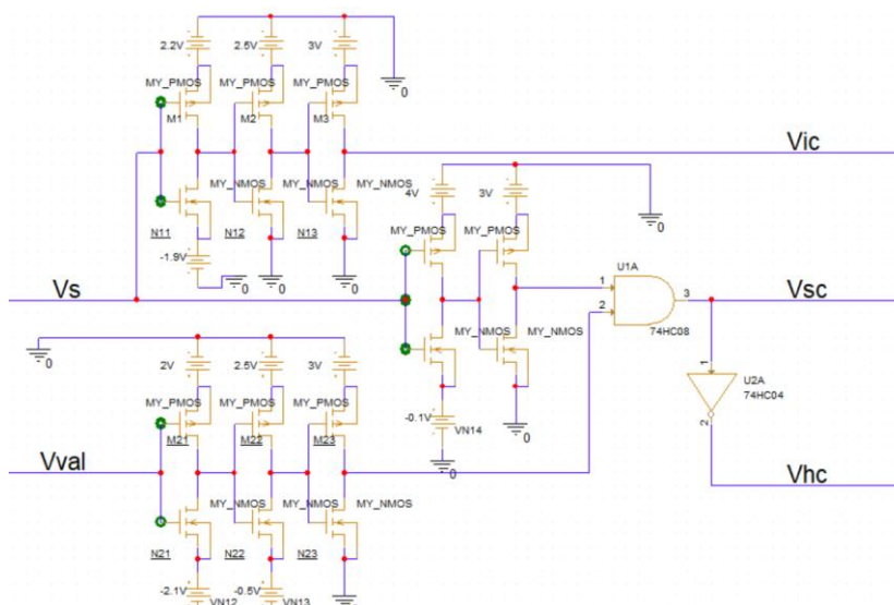
图 2-3 SJ单元电路图
