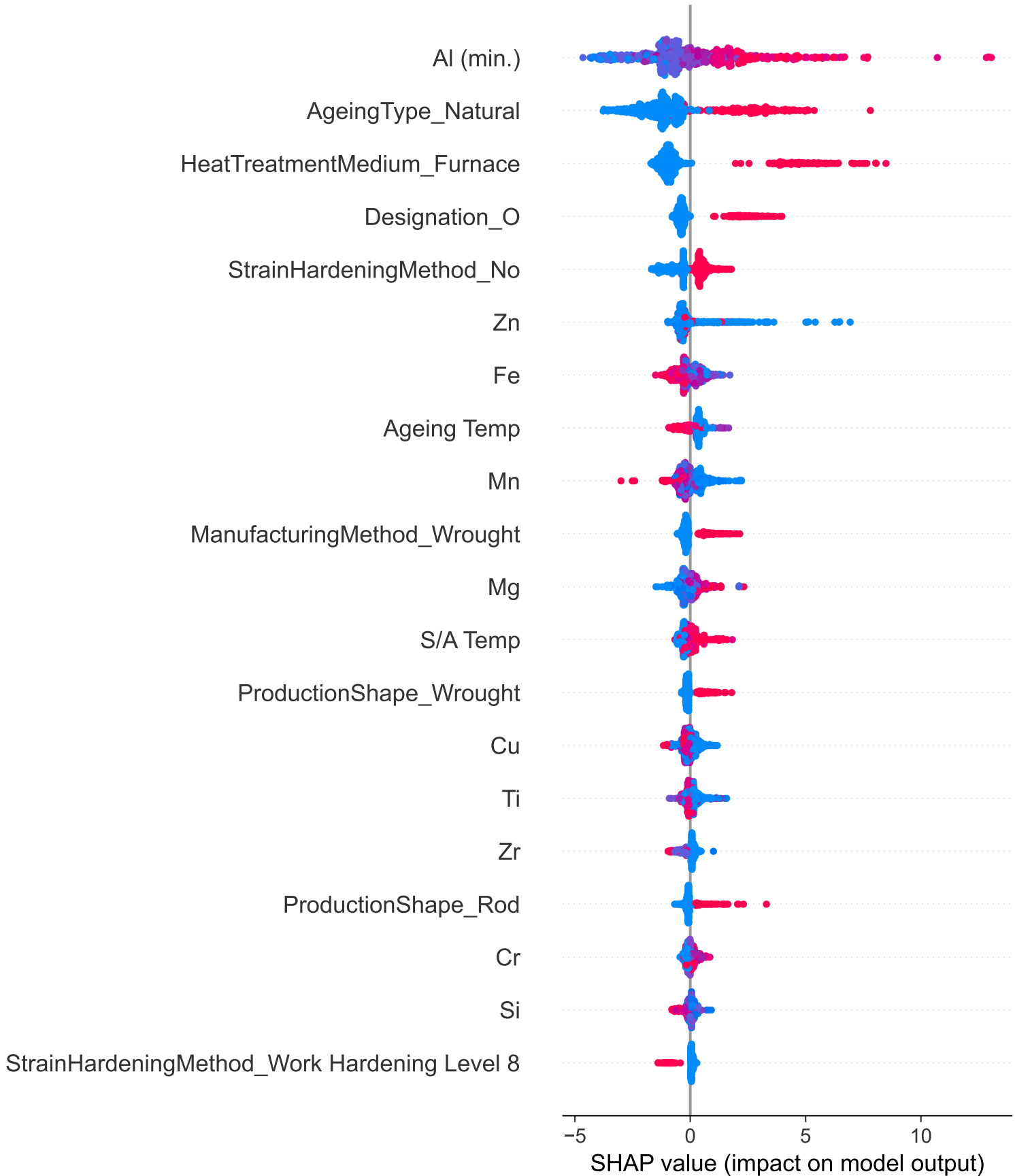
EL — SHAP Summary Plot
