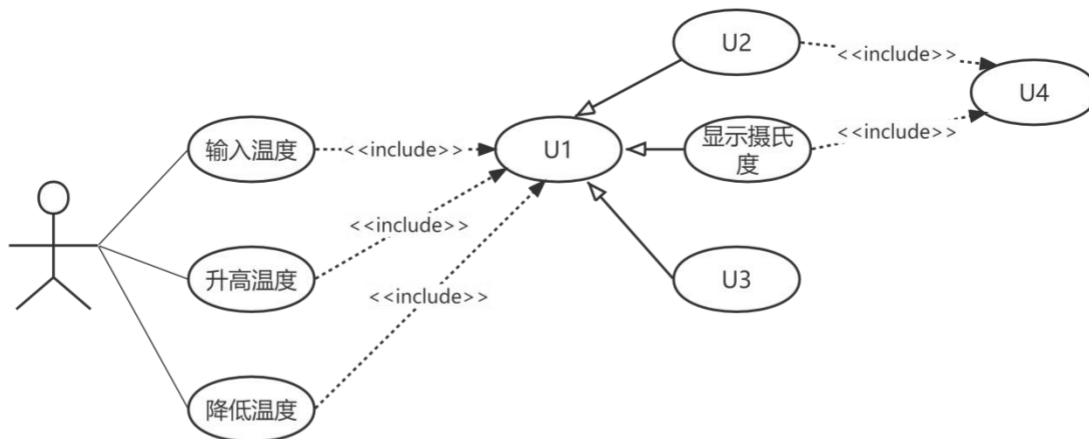
图3-2 用例图
