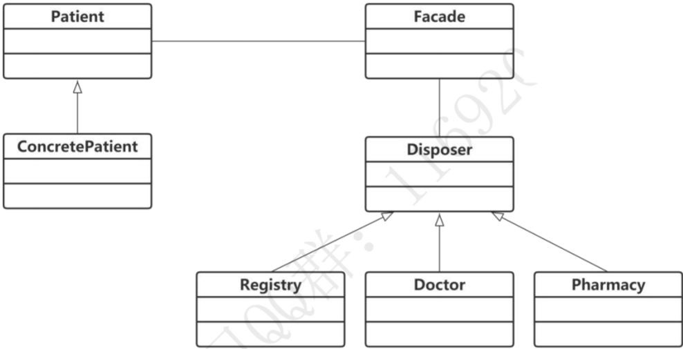
图5-1 类图
