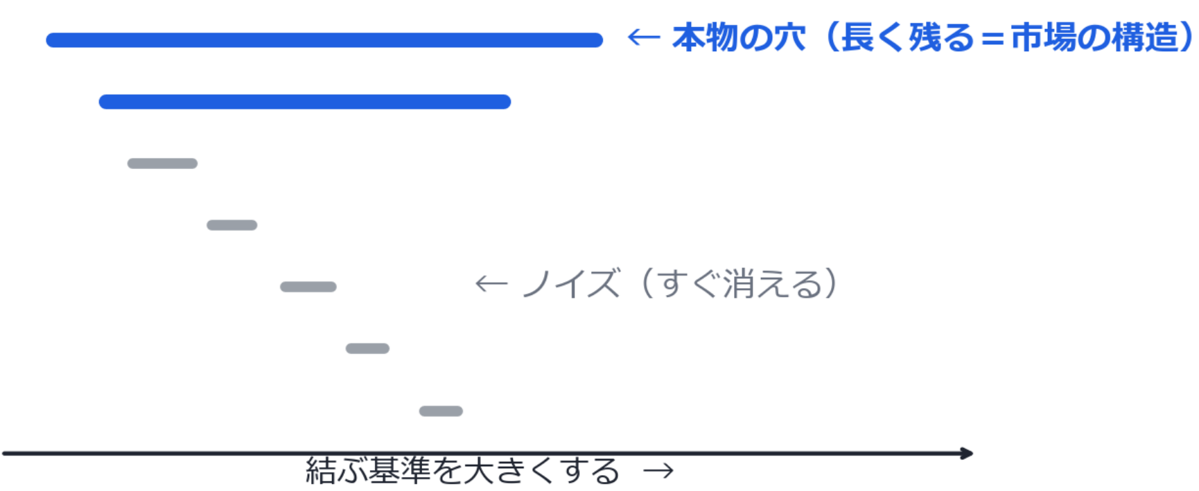
「近い点どうしを結ぶ基準」を大きくしていく →
