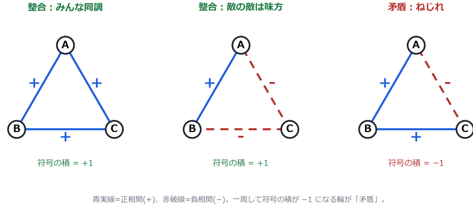
青実線=正相関(+), 赤虚線=負相関(-), 一周して符号の積が-1になる輪が「矛盾」。
