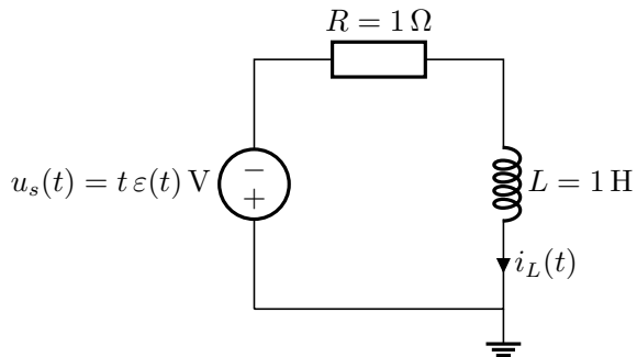
(a) 电路图
