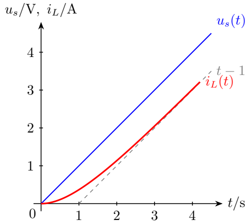
(b) 激励与响应波形
