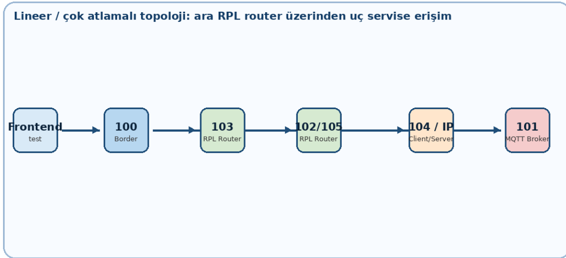
řekil 2. Lineer topoloji: ara RPL yönlendiriciler üzerinden çok atlamalı iletişim akışı.
