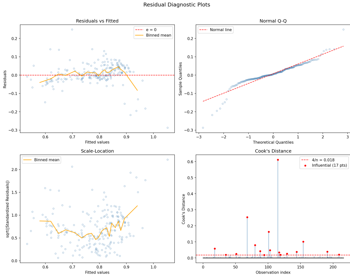
Hình 15: Bốn biểu đồ chẩn đoán phần dư của mô hình Lasso: Residuals vs Fitted, Normal Q-Q, Scale-Location và Cook's Distance.
