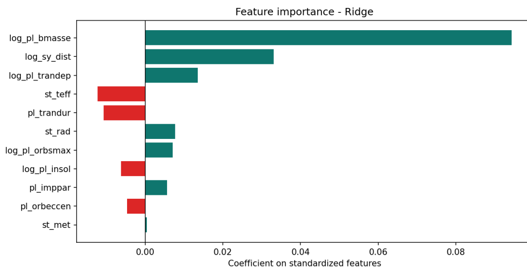
Hình 14: Feature importance dựa trên hệ số Ridge sau chuẩn hóa. Vì các feature đã được standardize, độ lớn hệ số có thể so sánh trực tiếp hơn.
