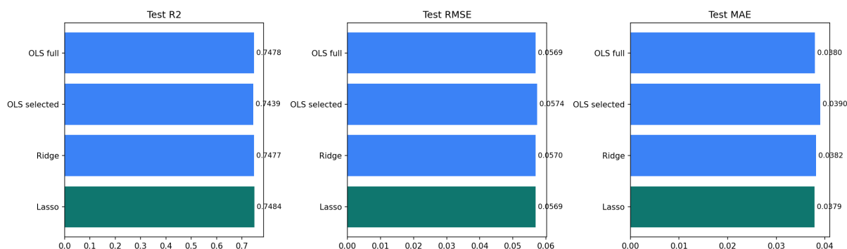
Hình 13: So sánh Test R^2 , RMSE và MAE giữa các mô hình tuyến tính. Lasso đạt Test R^2 cao nhất, nhưng khác biệt giữa Lasso, OLS full và Ridge rất nhỏ.
