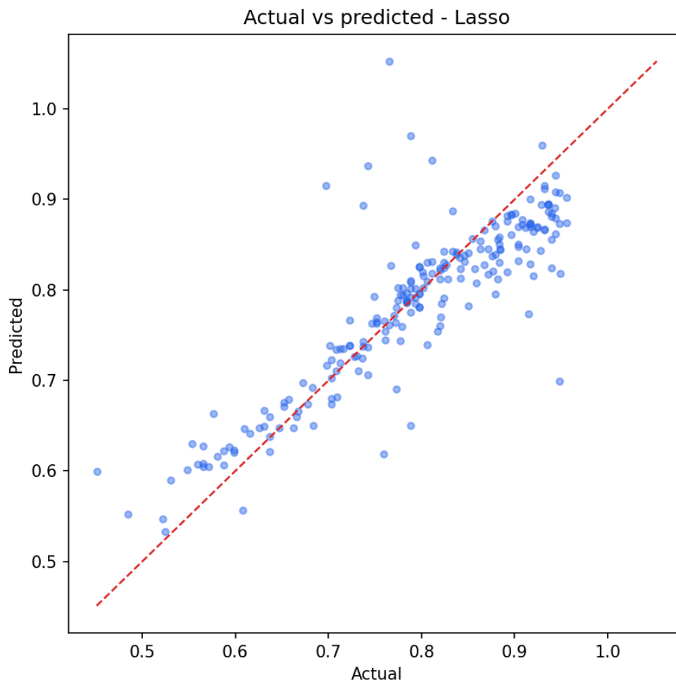
Hình 12: Actual vs Predicted trên tập test của mô hình Lasso. Các điểm càng gần đường chéo thì dự báo càng sát giá trị thật.
