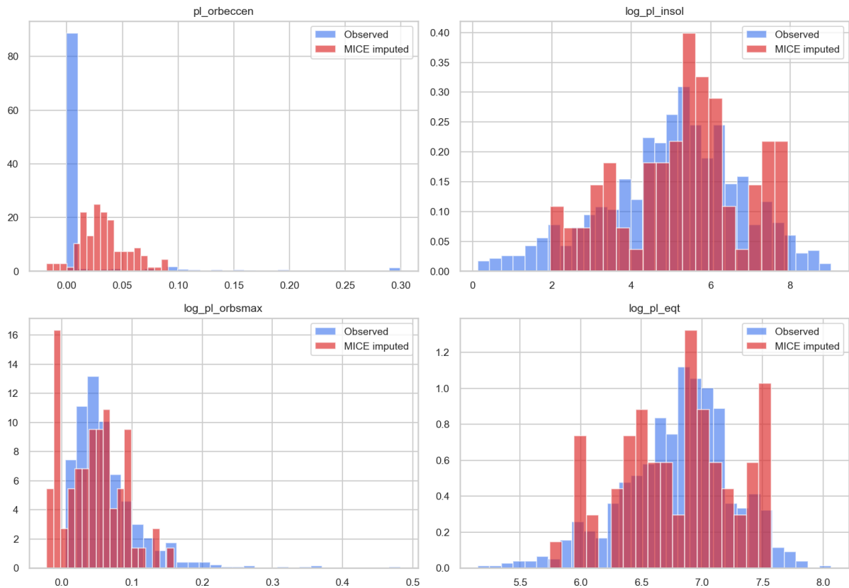
Hình 10: So sánh phân phối observed và phân được MICE impute. Giá trị impute không bị gom về một điểm trung vị duy nhất mà vẫn có độ phân tán theo quan hệ đa biến.
