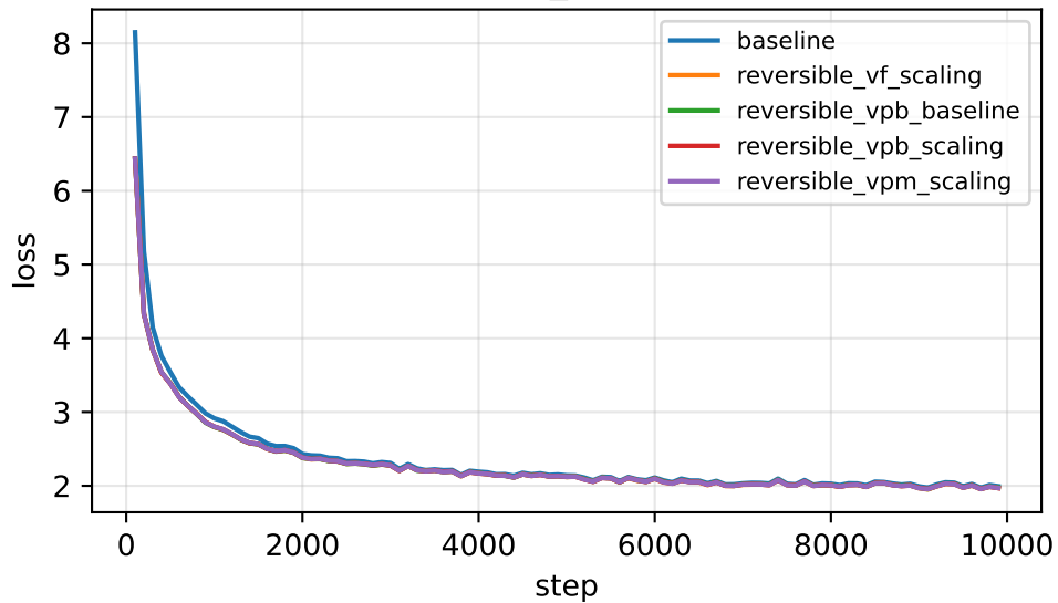
val_loss
