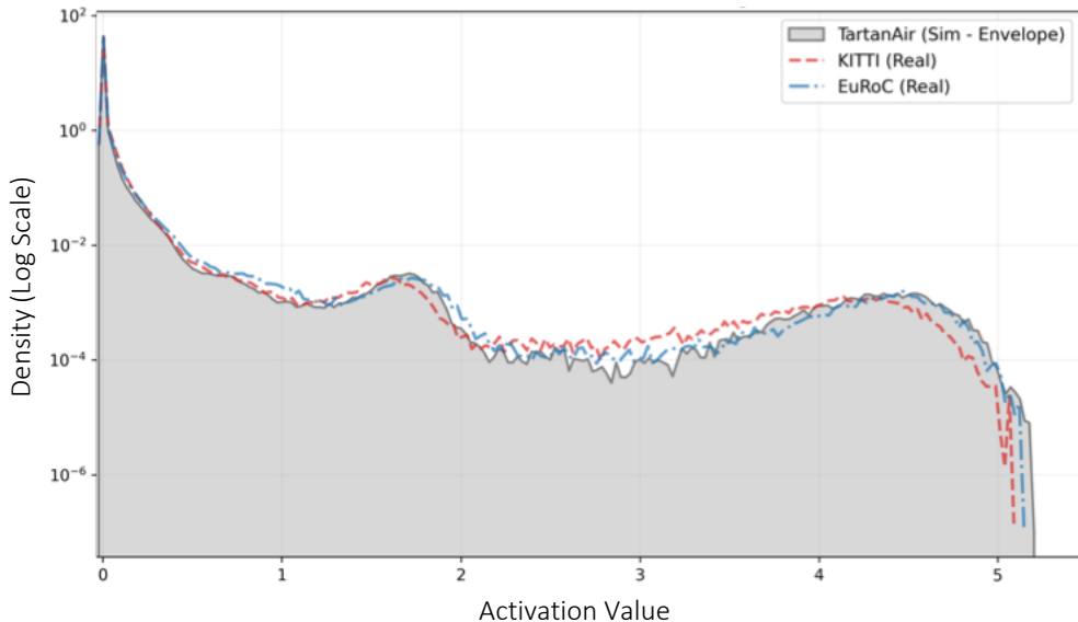
Layer: memory_decoder.cov_update.cov_head.conv4
