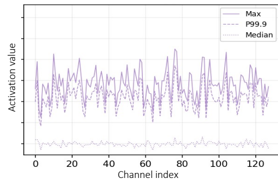
(d-1) Ours
